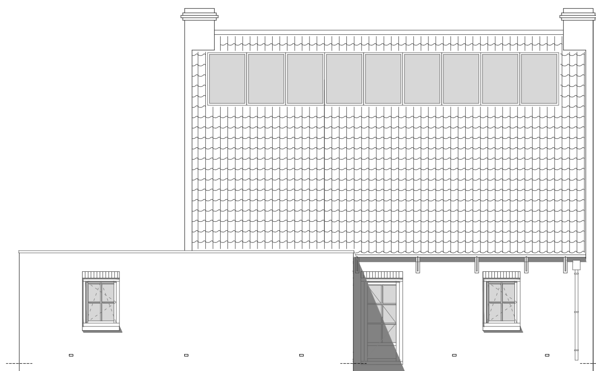
Oostgevel
