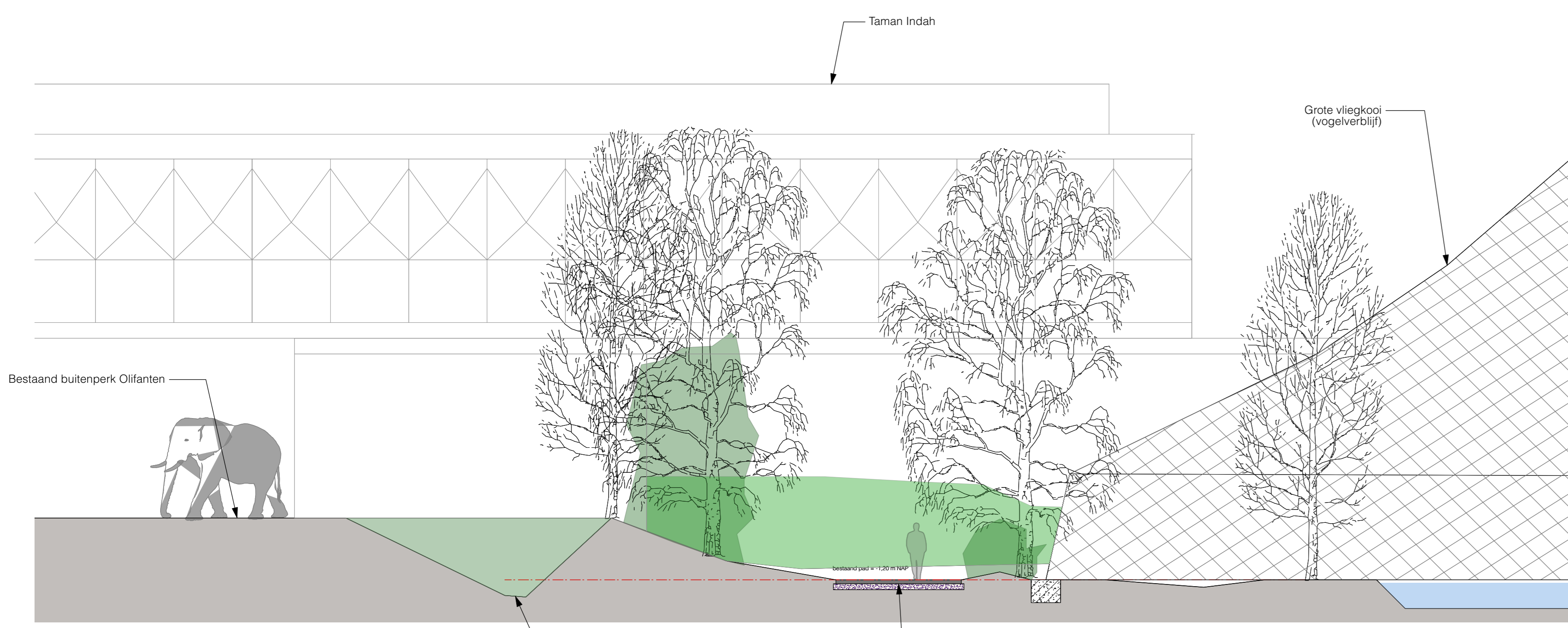
Doorsnede C-C ; Aanzicht vanaf pad zuidzijde
