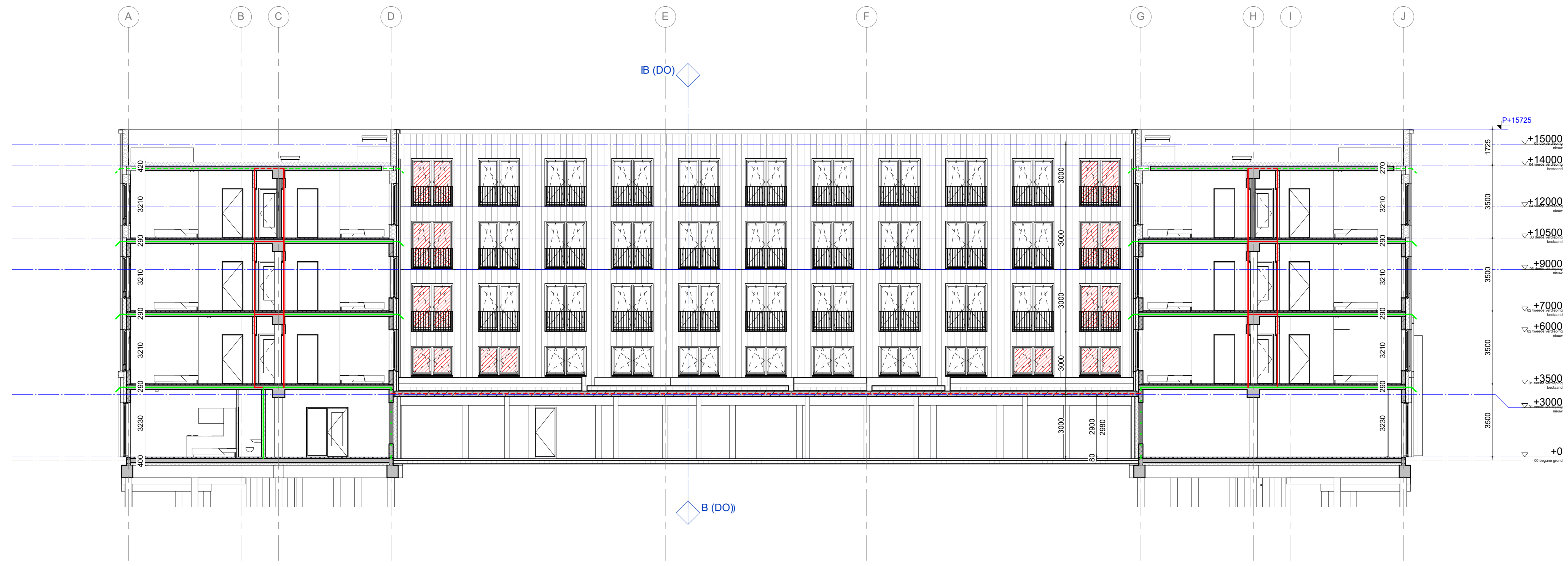
doorsnede A
