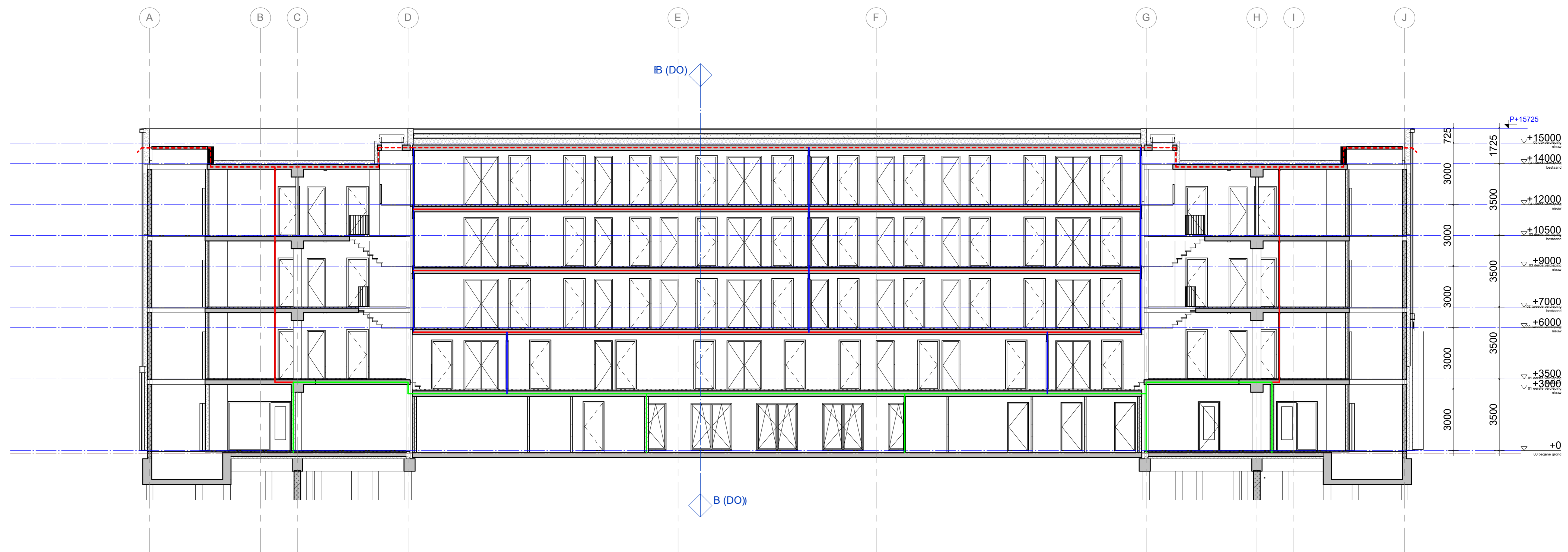
doorsnede C
