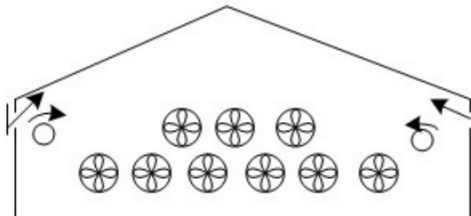
Doorsnede dwars
