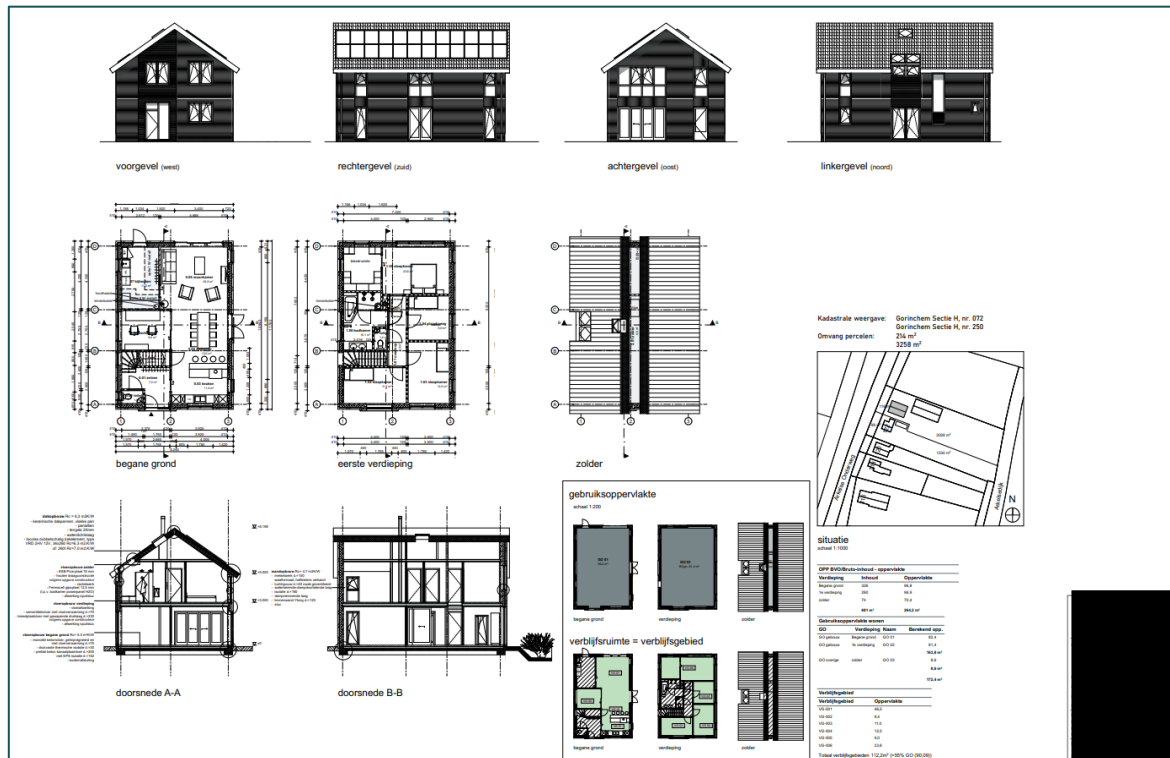
Figuur 1.4 Schetstekening van de beoogde woning (bron: Verhaar).
