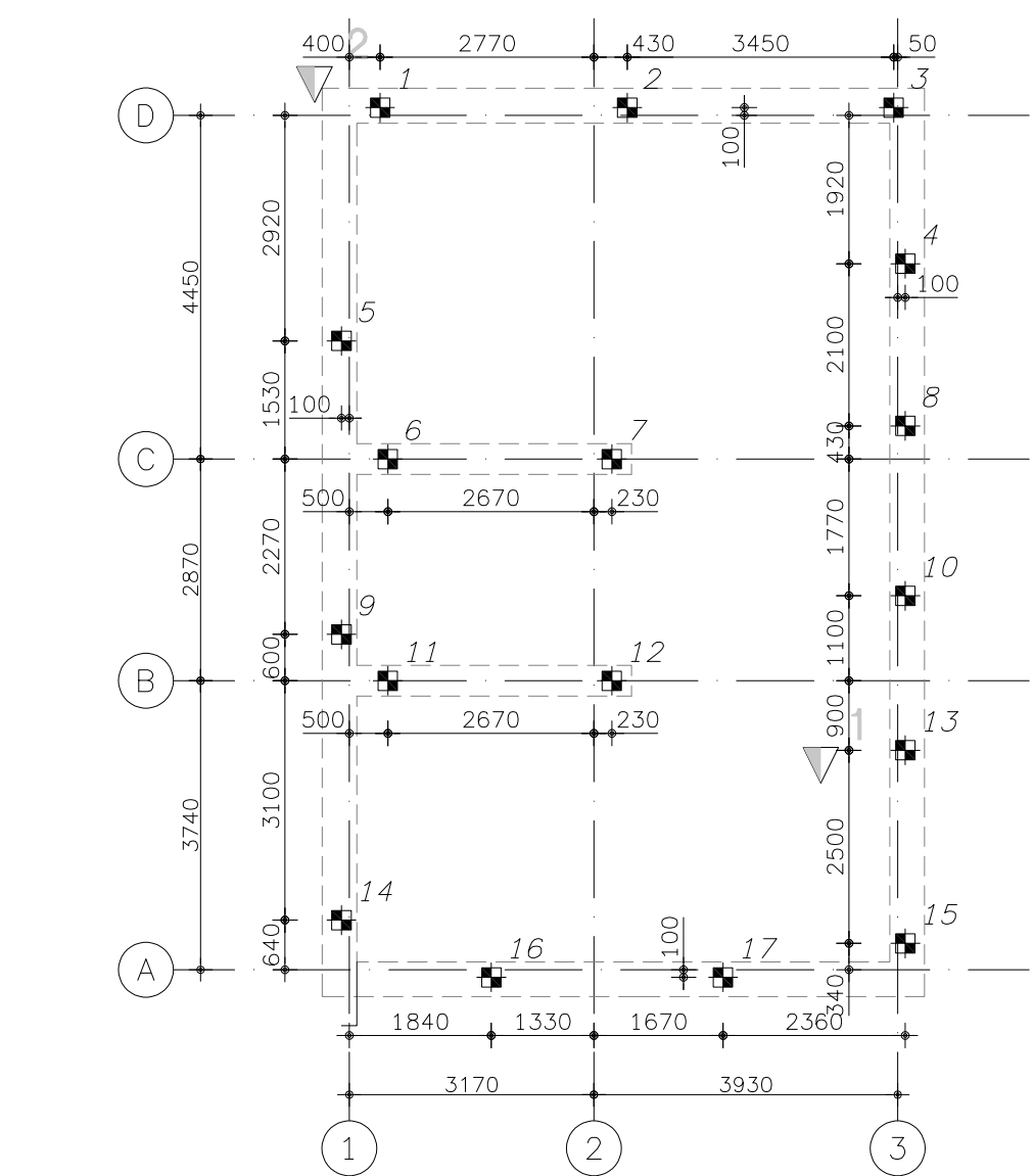
Palenplan
