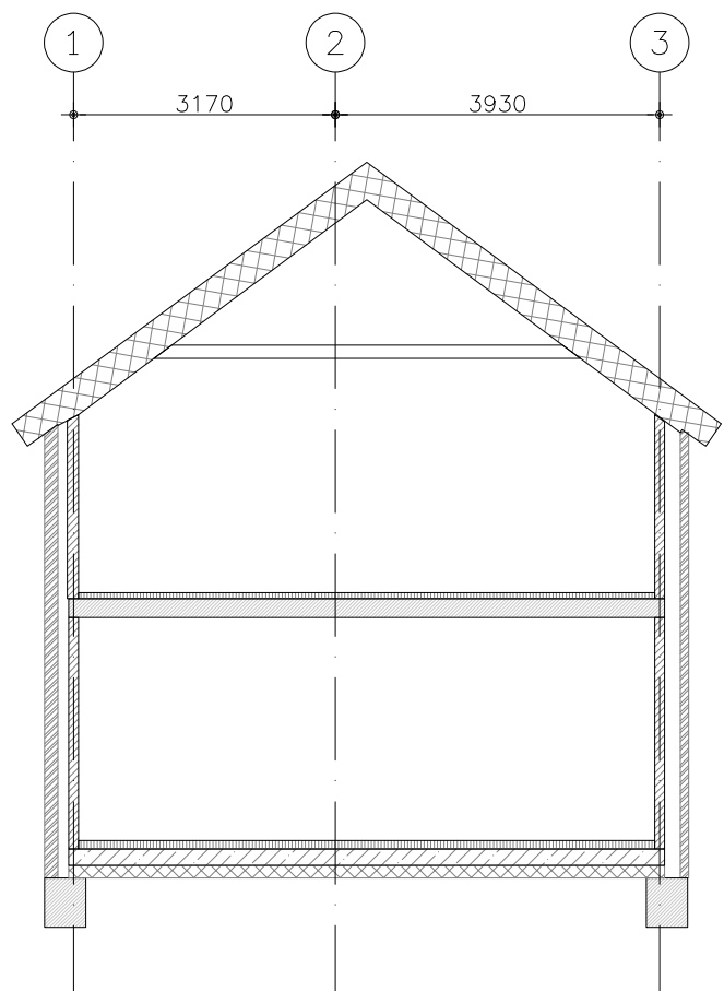
Doorsnede
