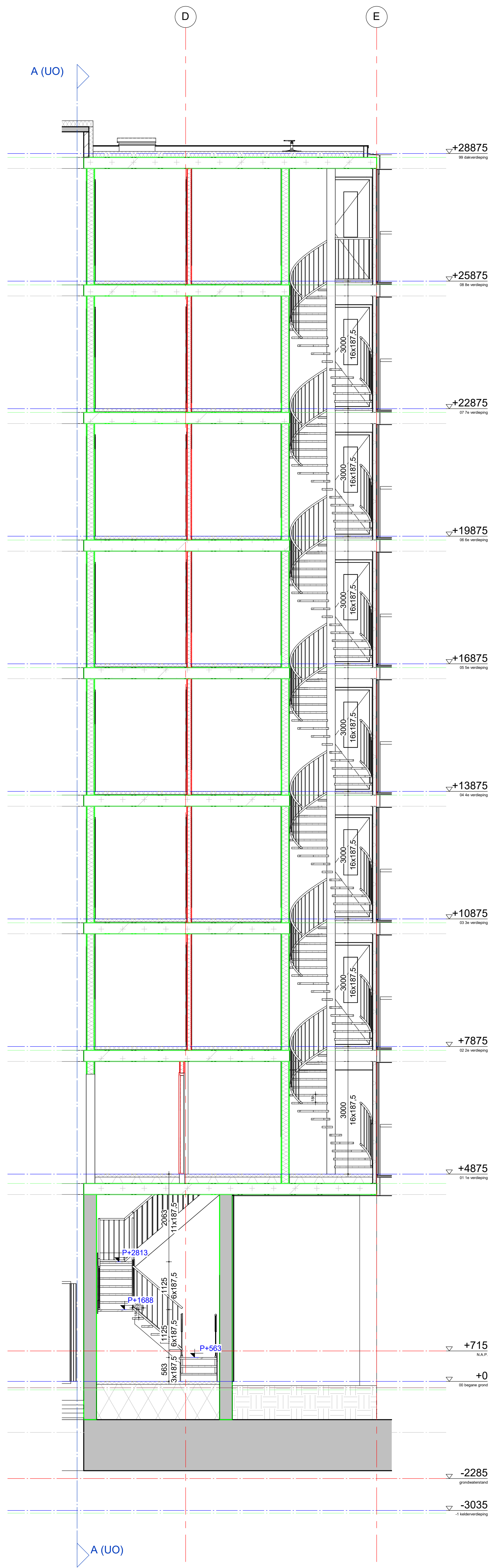
langsdoorsnede
