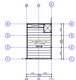
1e VERDIEPING 4000+ schaal 1:200
