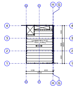
1e VERDIEPING 4000+ schaal 1:200
