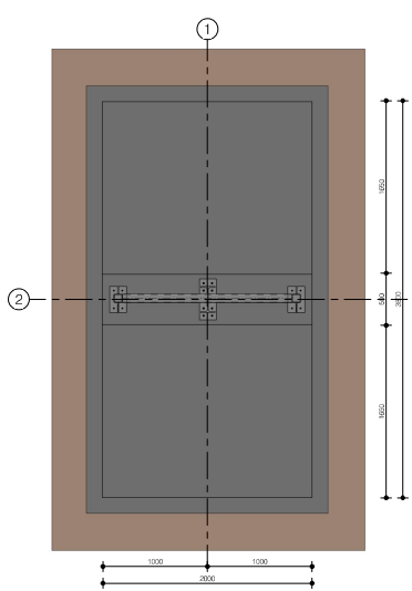
Maaielveld 1:30
