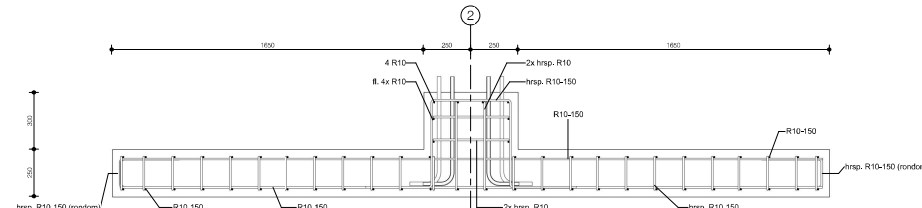
Wapening dwarsdoorsnede 1:30
