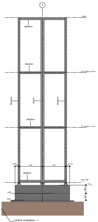
Zijaanzicht 1:30
