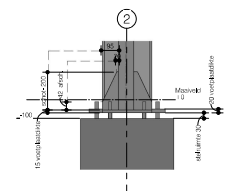
Detail voetplaten 1:30
