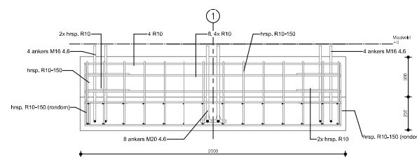
Wapening opstelling 1:30
