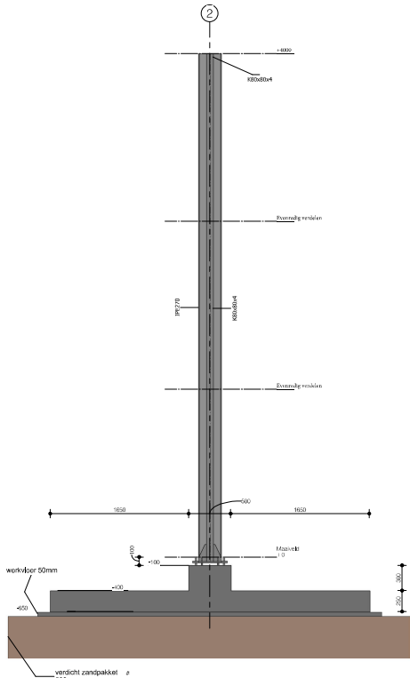
Vooraanzicht 1:30
