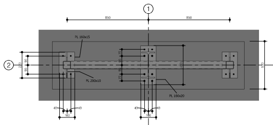
Voetplaten 1:30
