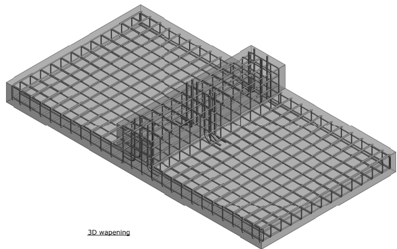
Voetplaten 1:30
