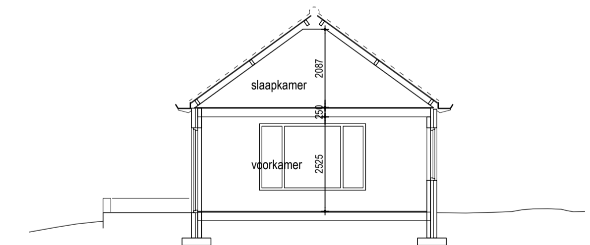
Dwarsdoorsnede
