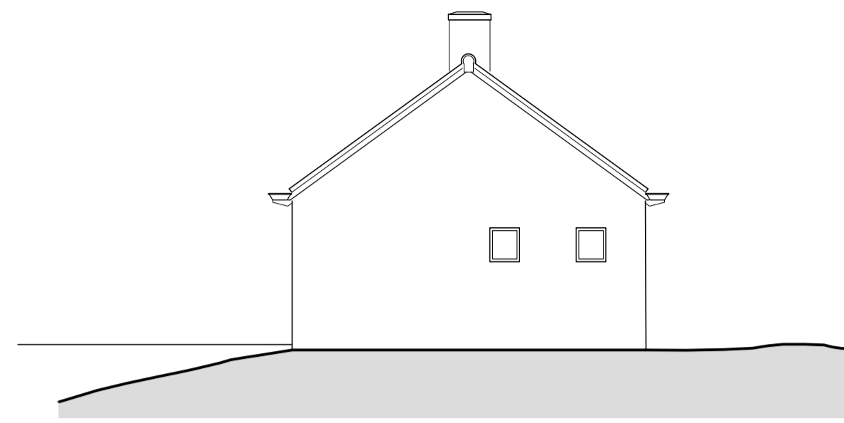
Noordoost gevel
