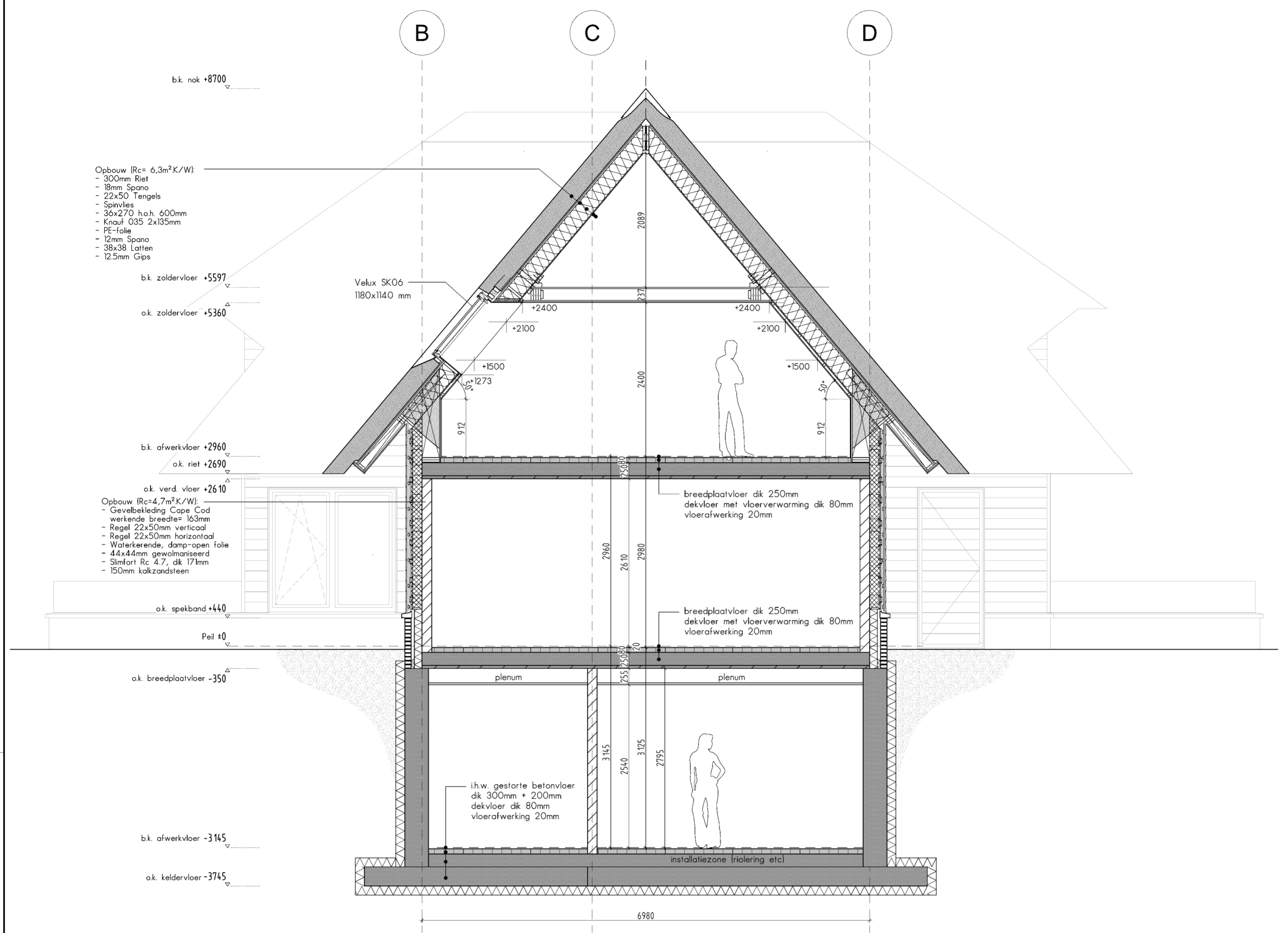
DOORSNEDE C-C
