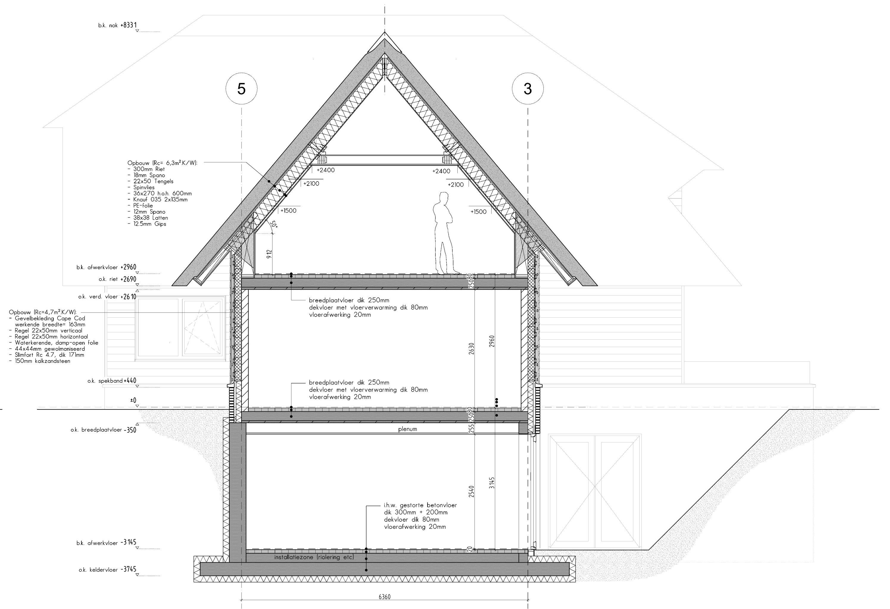
DOORSNEDE B-B
