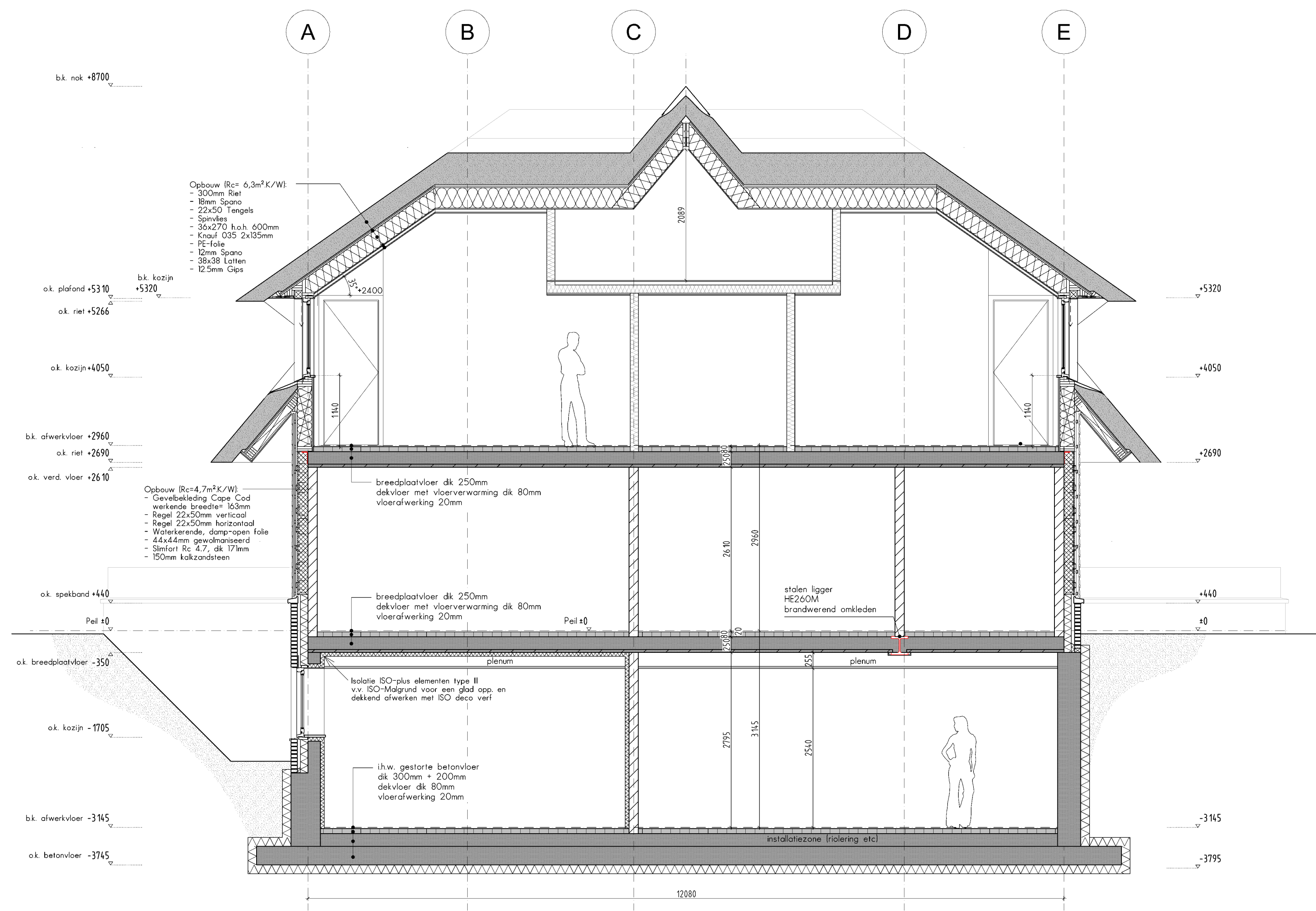
DOORSNEDE A-A
