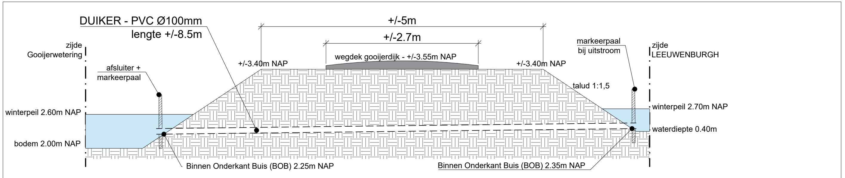
DOORSNEDE AA' 1:40
