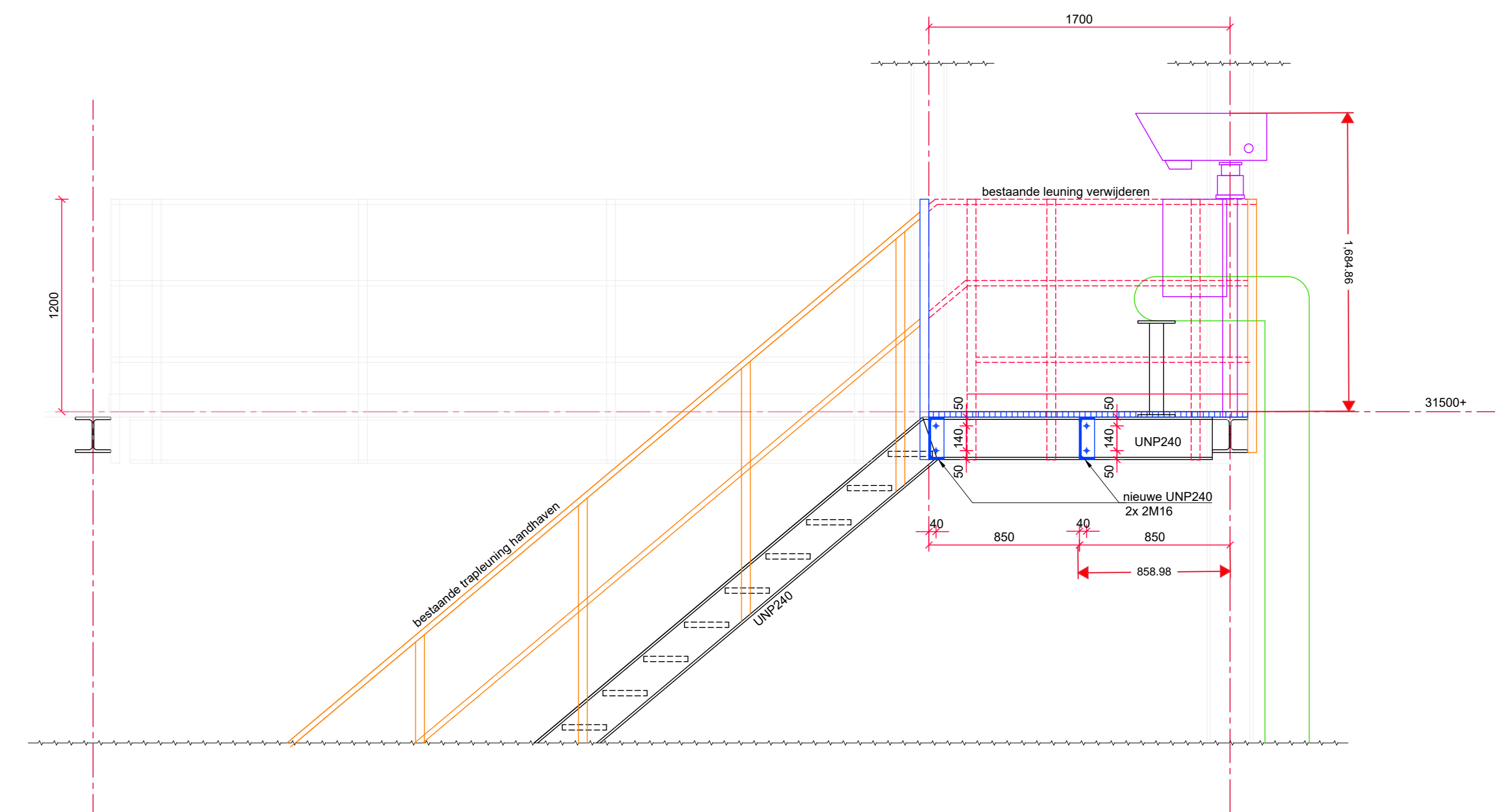
Doorsnede B-B
