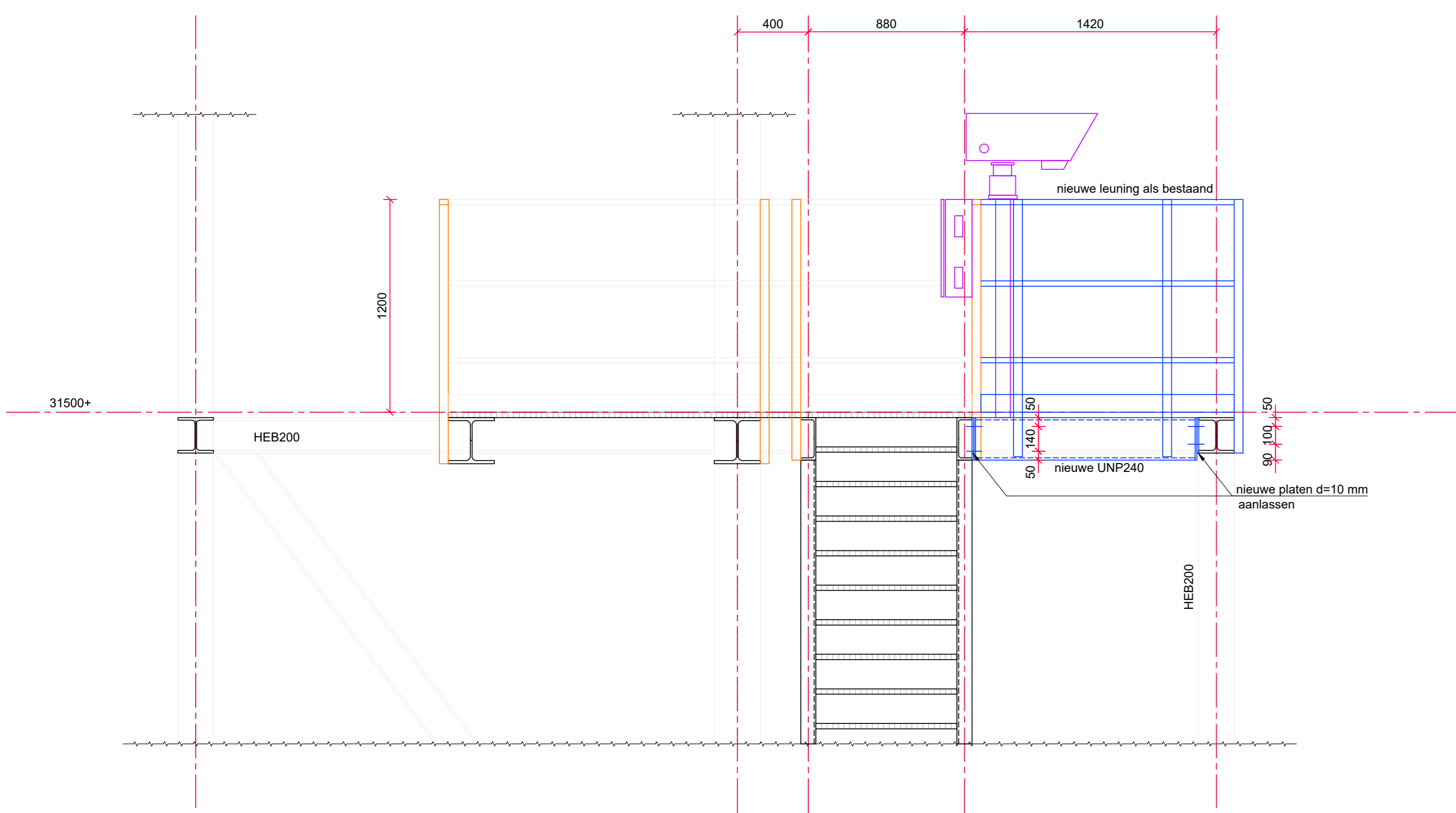
Doorsnede A-A
