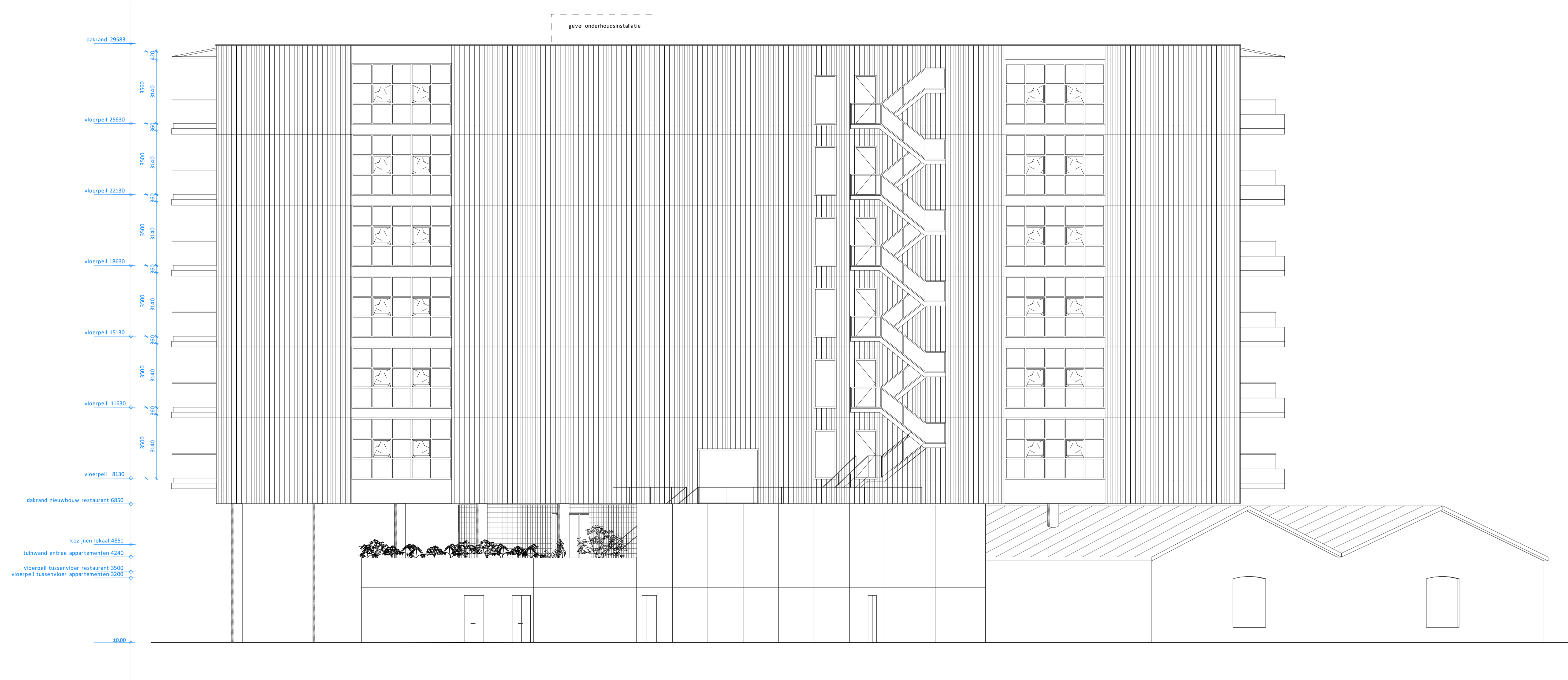
gevelaanzicht noordoost
