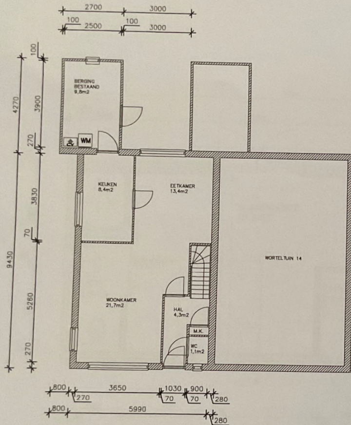
BEGANEGROND BESTAAND
