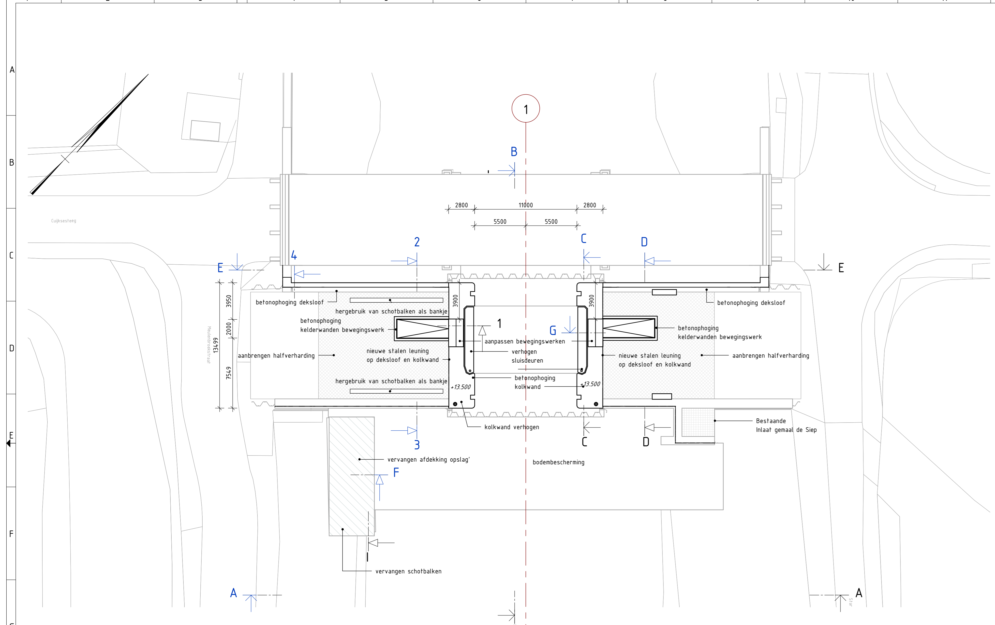
Bovenaanzicht schaal: 1 : 200
