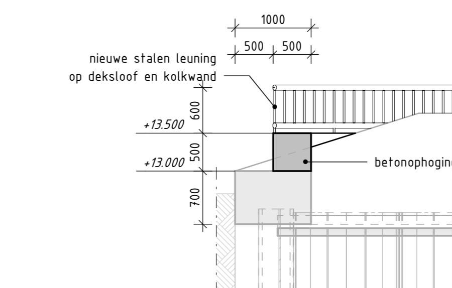
Detail 4 schaal: 1 : 50
