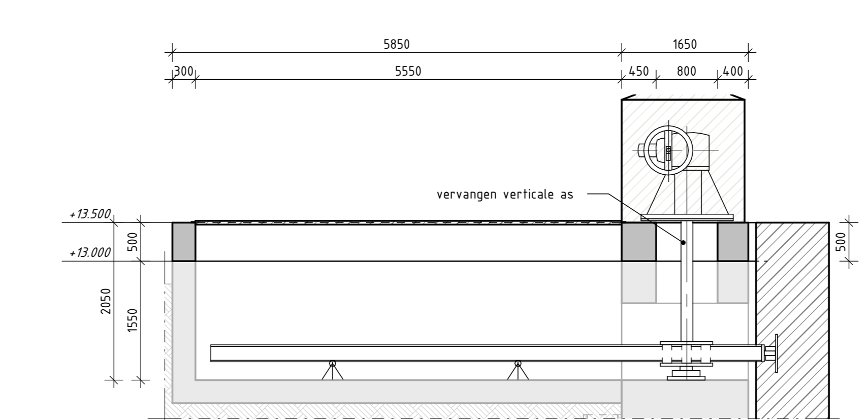
Detail 1 schaal: 1 : 50
