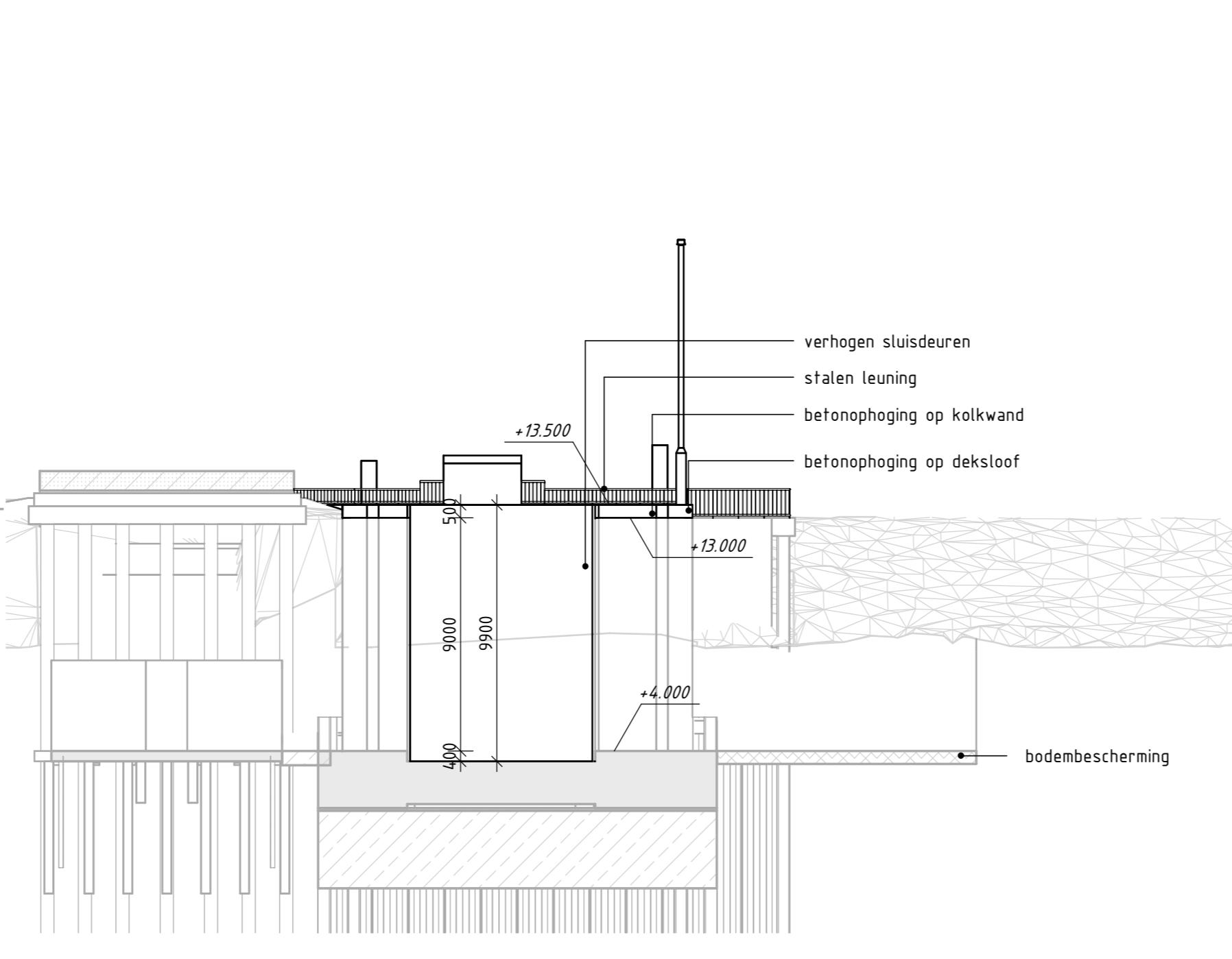
Doorsnede B-B schaal: 1 : 200
