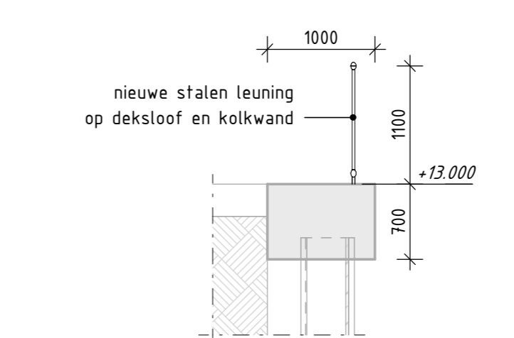
Detail 3 schaal: 1 : 50
