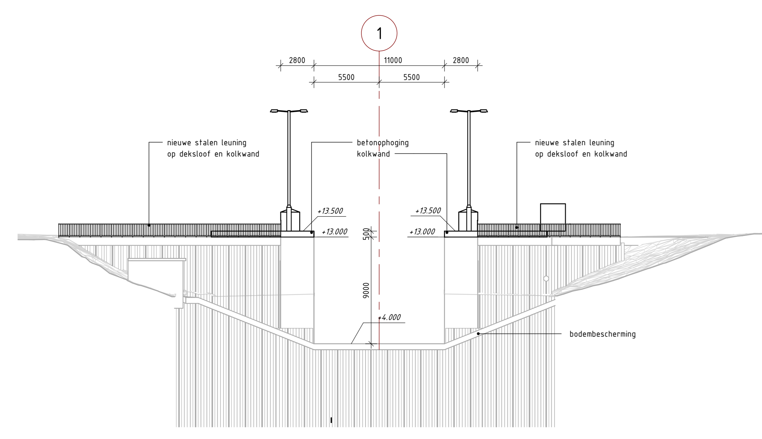
Aanzicht A-A schaal: 1 : 200
