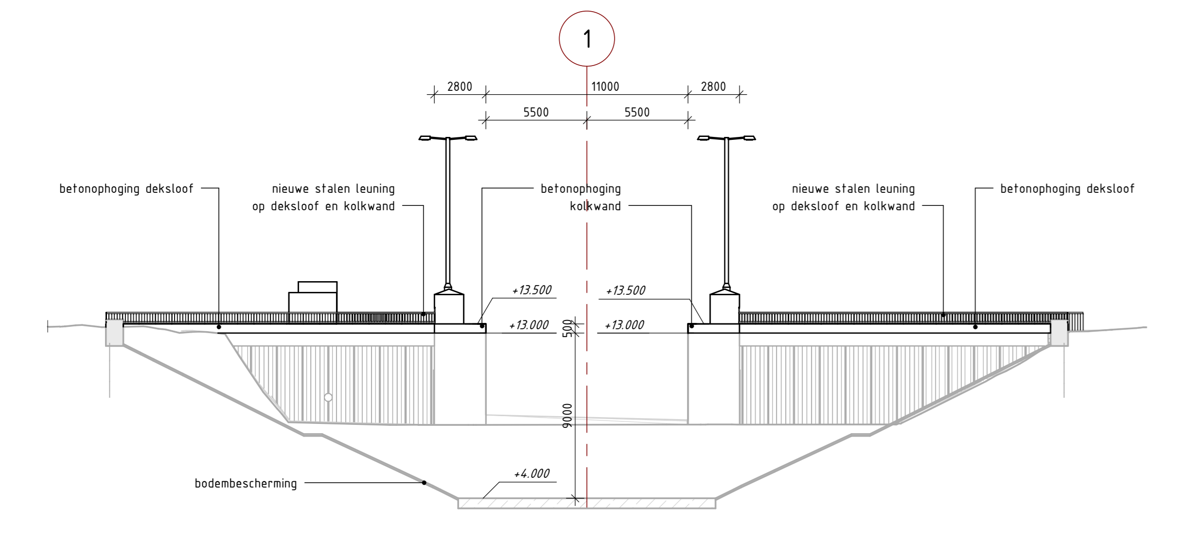
Aanzicht E-E schaal: 1 : 200
