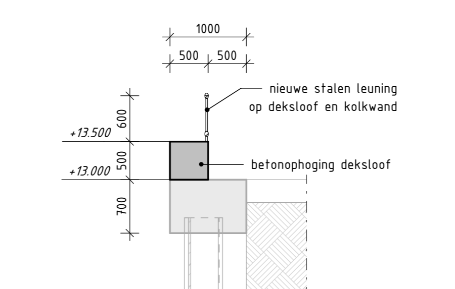
Detail 2 schaal: 1 : 50
