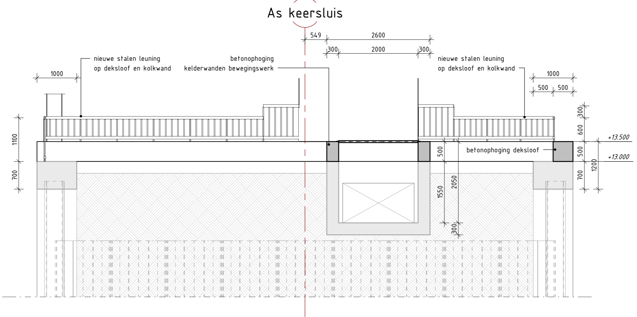
Doorsnede D-D schaal: 1 : 50
