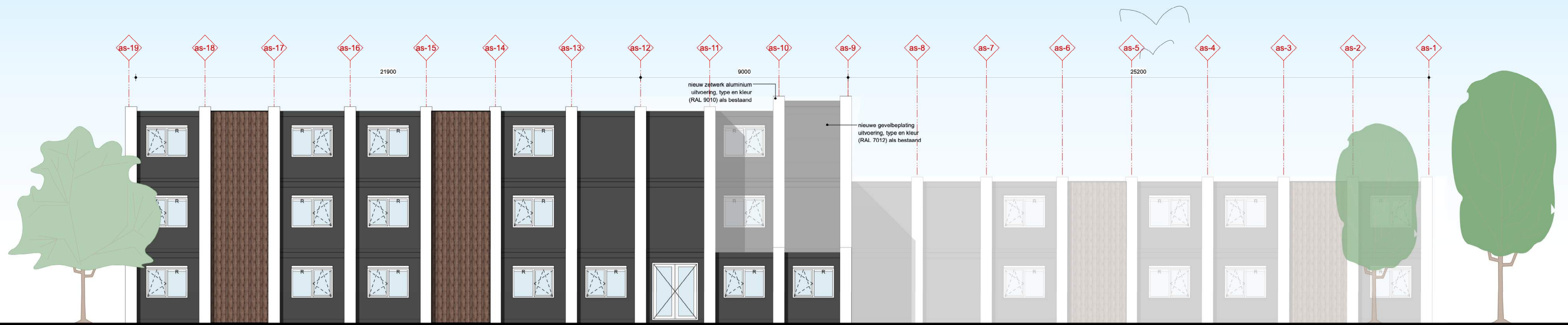
NOORDOOST GEVEL
