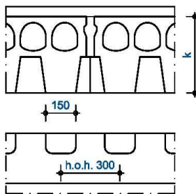
AANZICHTEN RANDOPLEGGING
