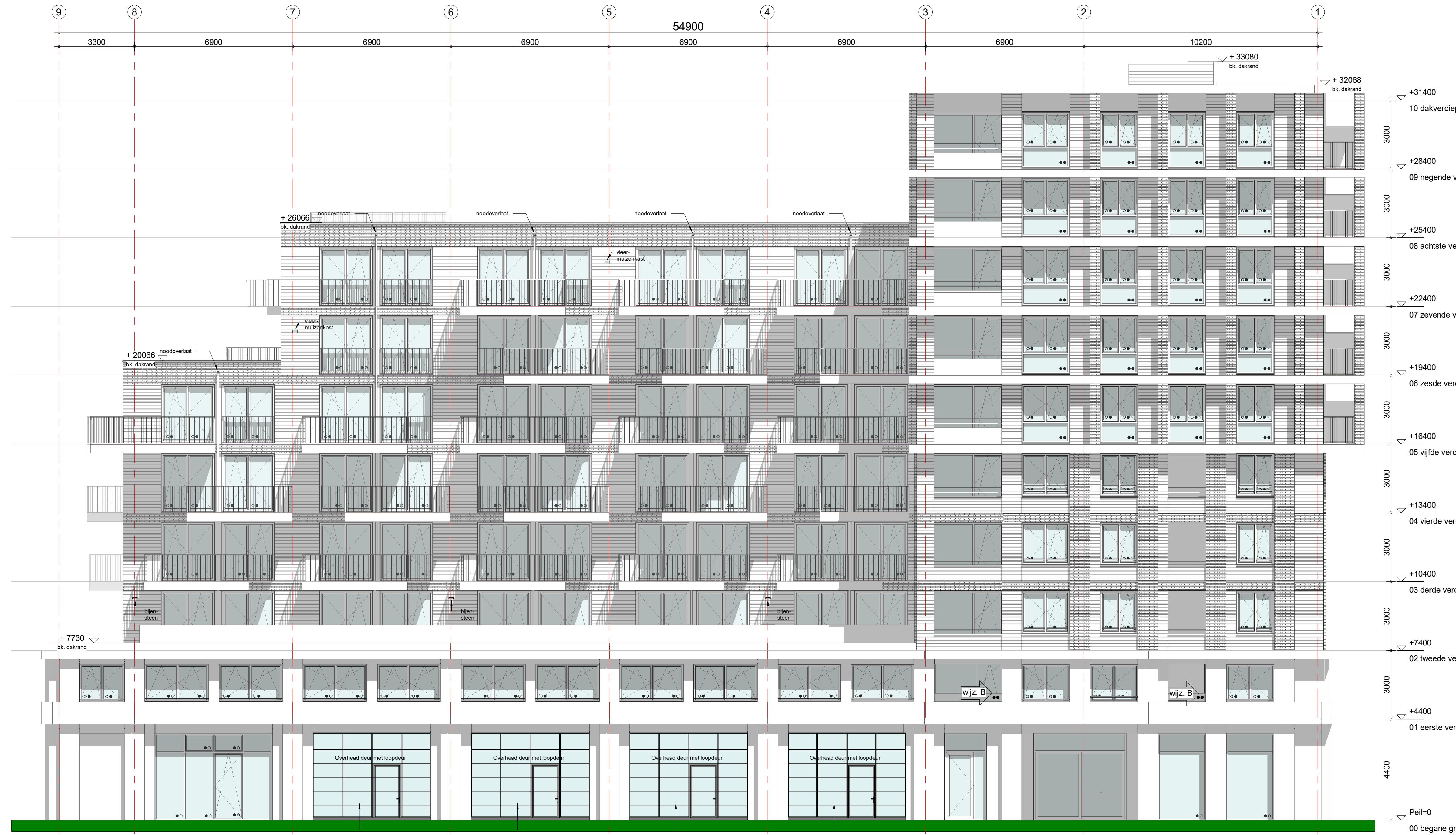
voorgevel Schoterbosstraat 1 : 100
