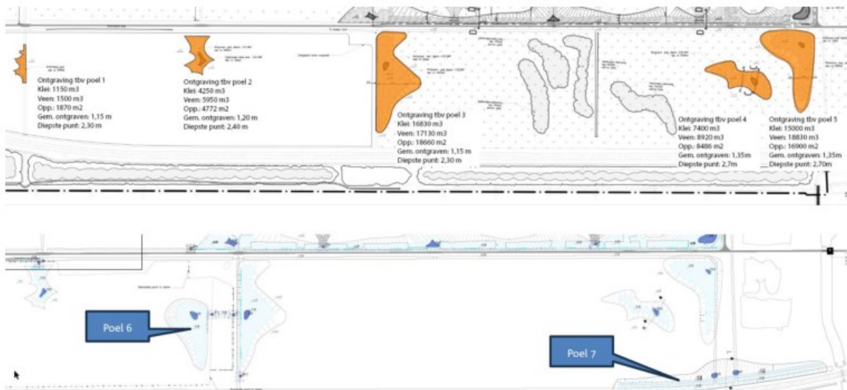
Figuur 2: Het graven van twee nieuwe poelen die in de vergunning van Z2019-0003033/D2020-149791 zijn aangewezen.
