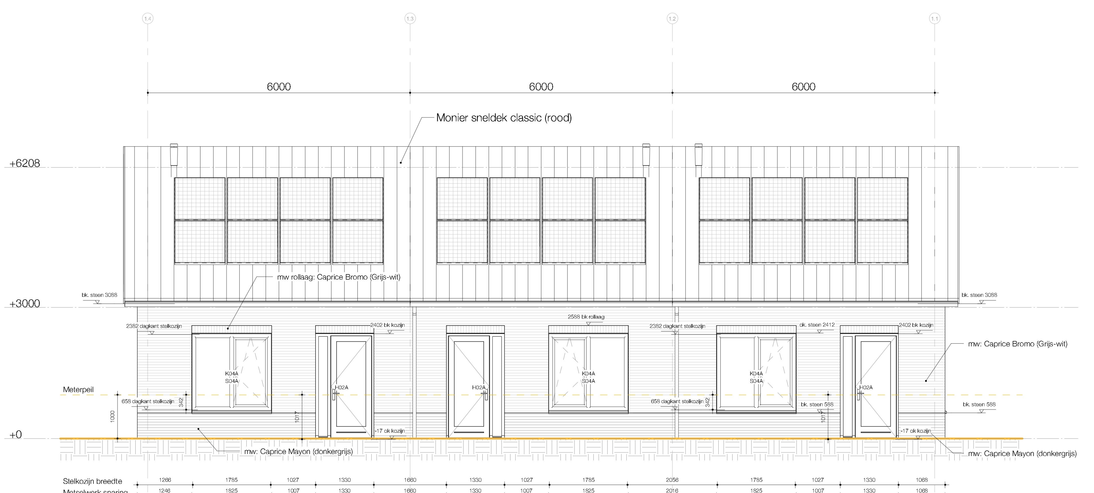
ACHTERGEVEL
