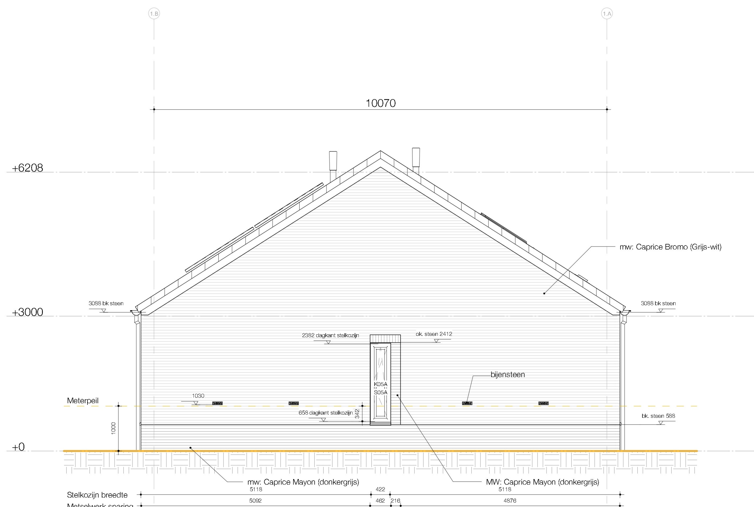
LINKER GEVEL
