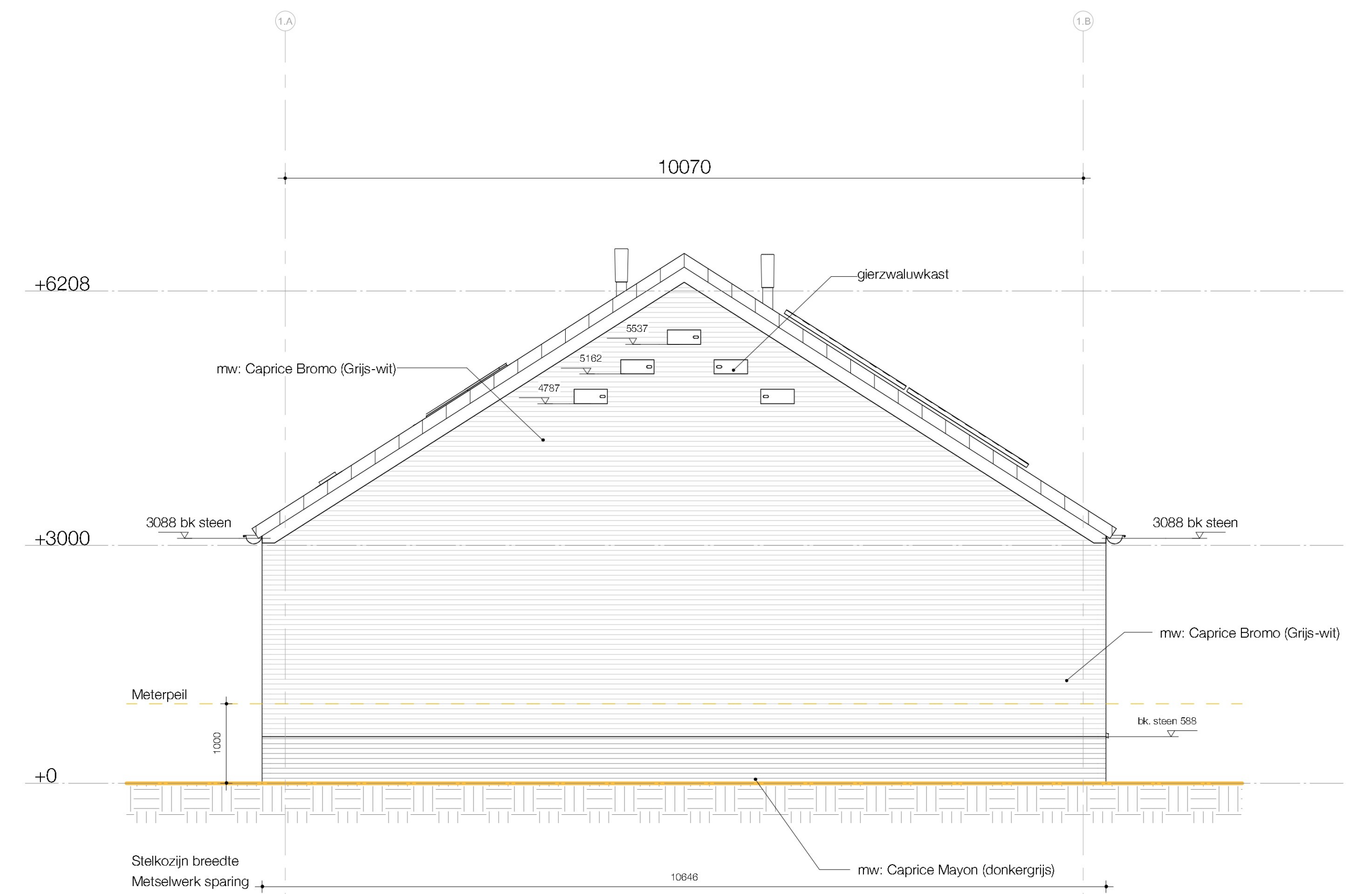
RECHTER GEVEL
