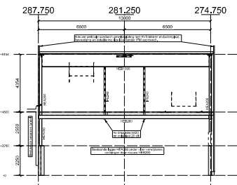
Aanzicht as-163.000 1:100
