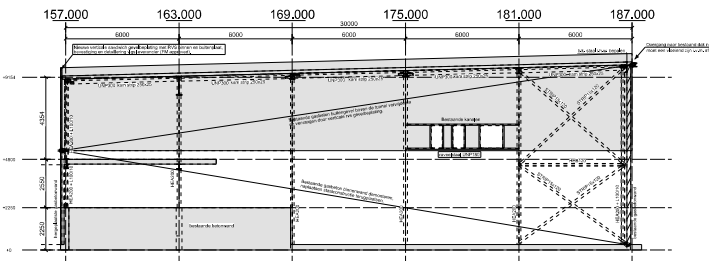
Aanzicht as-287.750 1:100
