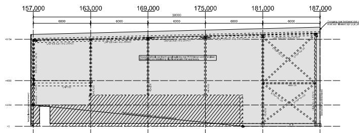
Aanzicht as-274.750 1:100
