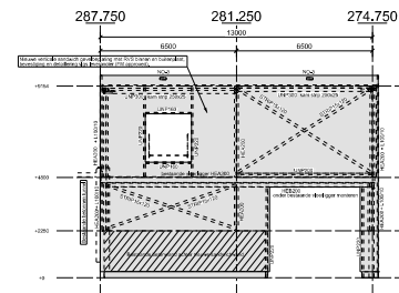
Aanzicht as-157.000 1:100
