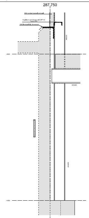
Nieuwe situatie linker zijgevel, boven betontunnel 1:10
