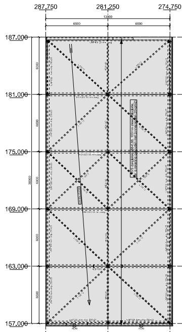
Dakvlak 1:100
