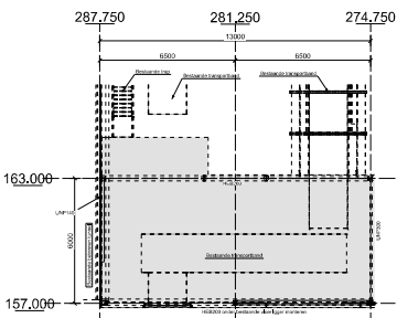
Verdiepingsvloer 1:100
