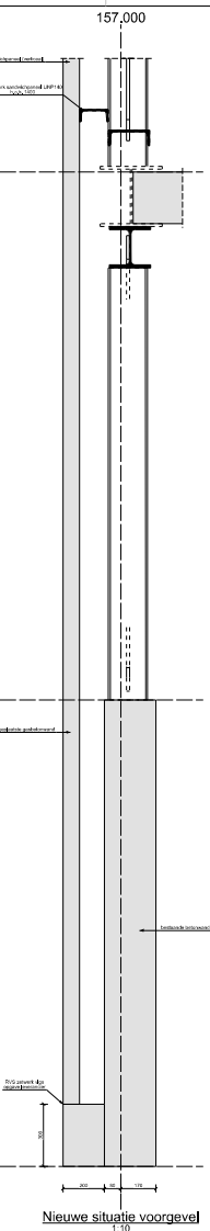
Nieuwe situatie linker zijgevel 1:10
