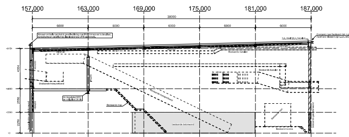
Aanzicht as-281.750 1:100
