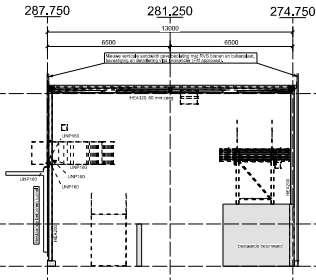
Aanzicht tussen stralmen 175.000 en 181.000 1:100
