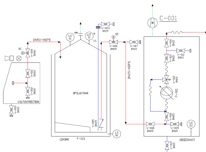
Figuur 1; Schematische weergave van de waterzuiveringsinstallatie
