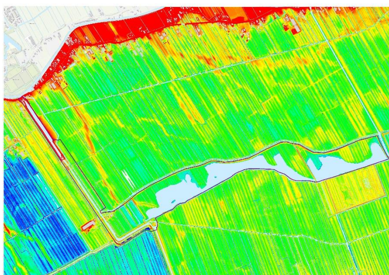
Figuur 8 Maaiveldhoogte plangebied (gebaseerd op Actueel Hoogtebestand Nederland (AHN4))
