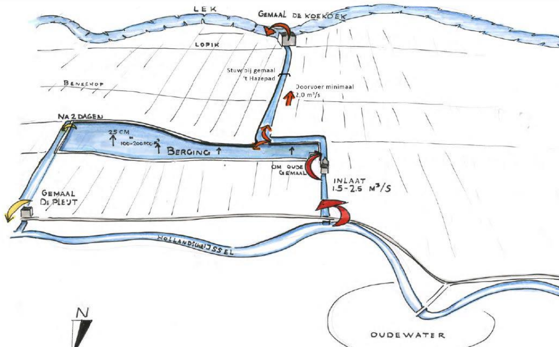
Figuur 6 Gewenste situatie wanneer gebruik wordt gemaakt van de waterberging of de doorvoermogelijkheid
