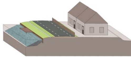
I 1b: Ophoging rijbaan i.c.m. bodemverzwaring
