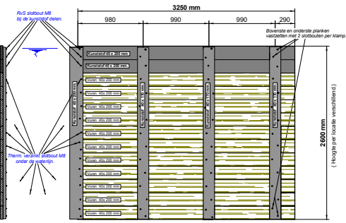
Samengesteld Beschoeiingsschot. 260 cm hoog met 2 kunststof planken. Klamps en delen bevestigen met schroeven.
