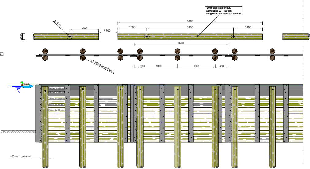
Voorbeeld: Golfbreker met opgeklampt schot tot in de Bodem.
