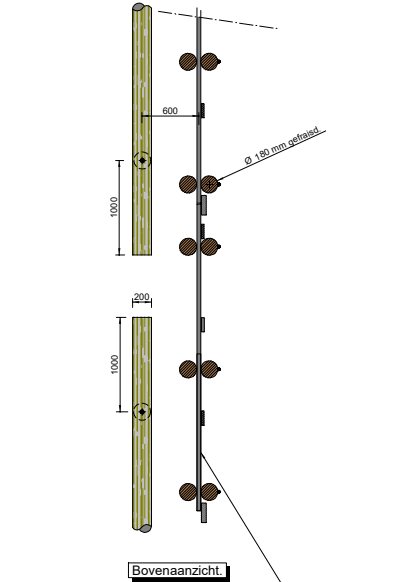
Samengesteld Beschoeiingsschot. 260 cm hoog met 2 kunststof planken. Klamps en delen bevestigen met schroeven.
