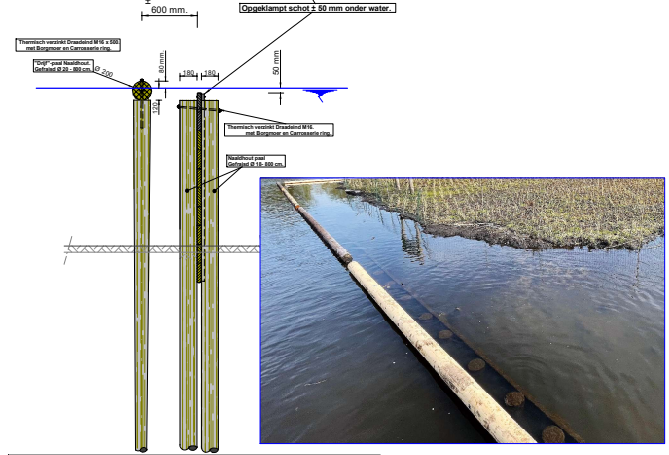
Opstelling schot ± 50 mm onder water met drijfbalk.
