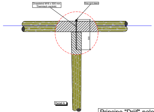
Principe "Drijf"-palen.
