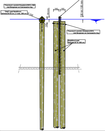
Opstelling schot ± 100 mm boven water met drijfbalk.
