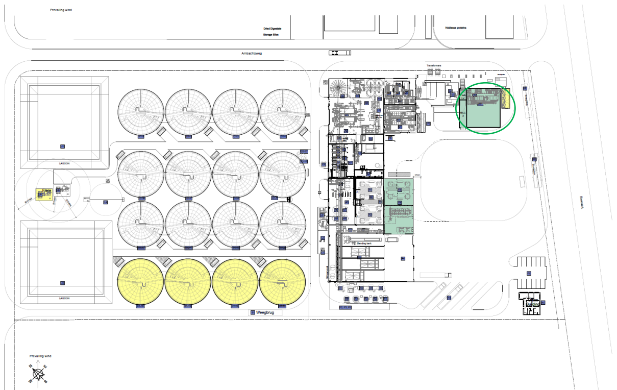
Figuur 3 plattegrond van de inrichting met daarop aangegeven de positie van het nieuwe gebouw voor de groen gas opwerkinstallaties (groen omcirkeld). Zie ook bijlage 2a bij de aanvraag voor gedetailleerde plattegrond.
