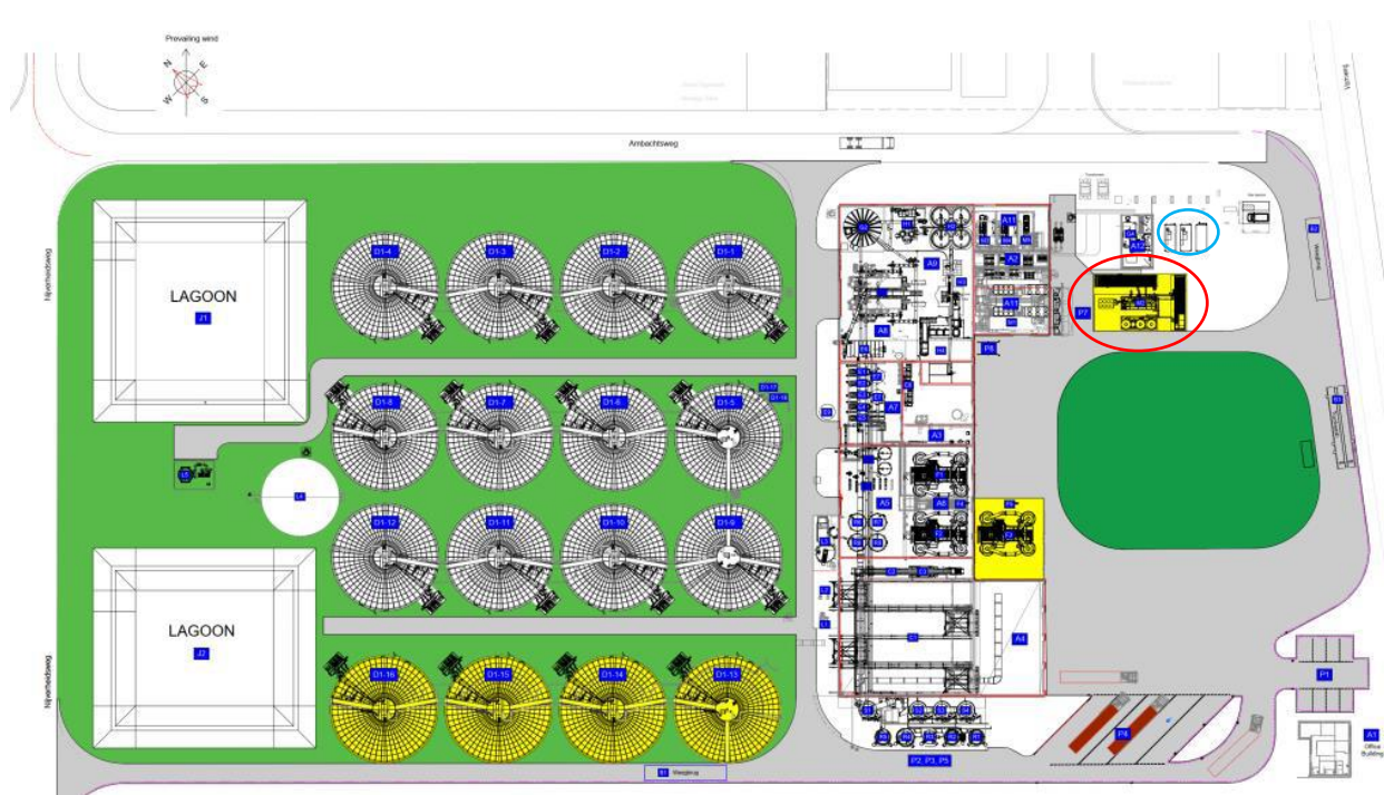
Figuur 2 Plattegrond inrichting met de vergunde groen gas opwerkinstallaties van 25 oktober 2022 (rood omcirkeld) en eerder (blauw omcirkeld)
