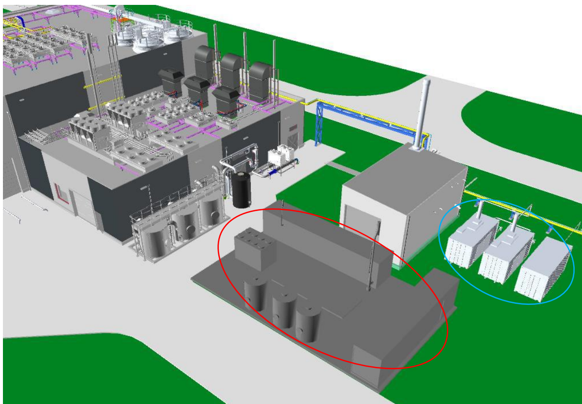
Figuur 1 Vergunde buitenopstelling extra groen gas opwerkinstallatie van 22 oktober 2022 (rood omcirkeld), en de al eerder vergunde groen gas opwerking (blauw omcirkeld)
