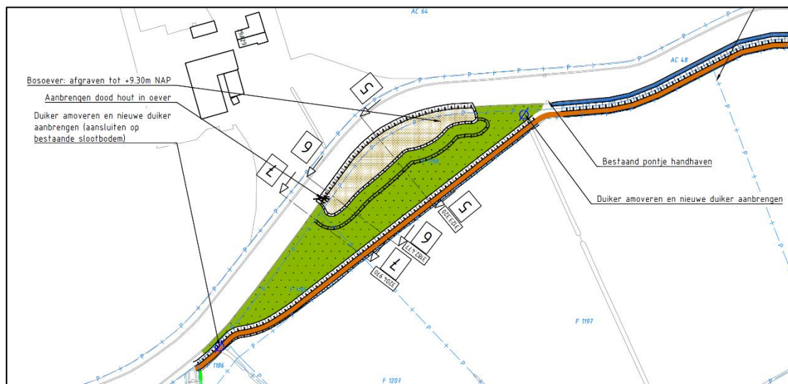
Figuur 3.7: Uitsnede ontwerp nabij Staringkoepel
