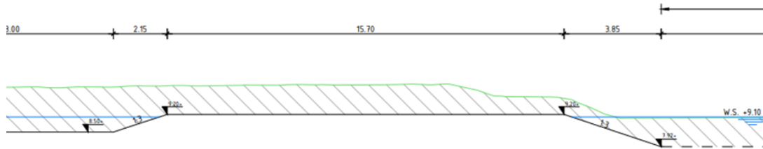
Figuur 3.6: Principeprofiel bosoever nabij pontje Staringkoepel (linkeroever)
