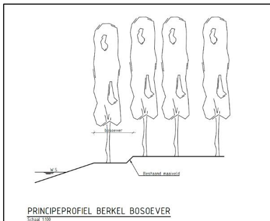
Figuur 3.5: Principeprofiel bosoever (niet vergraven)
