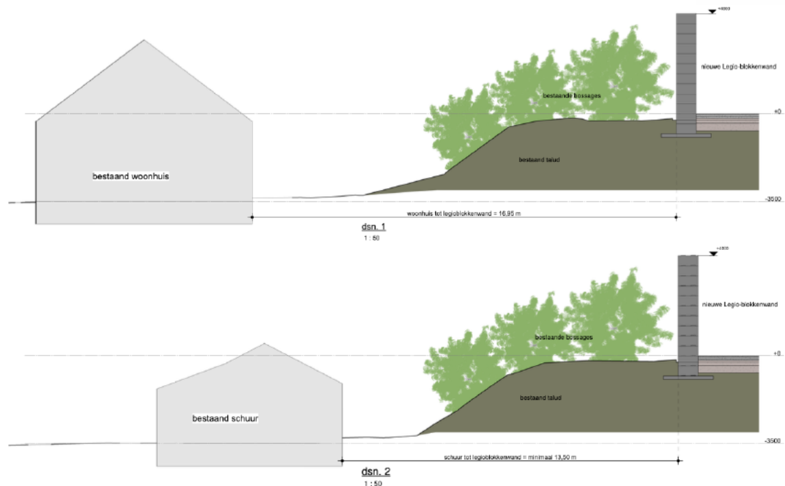
Figuur 2: positie keerwanden t.o.v. naastgelegen percelen
