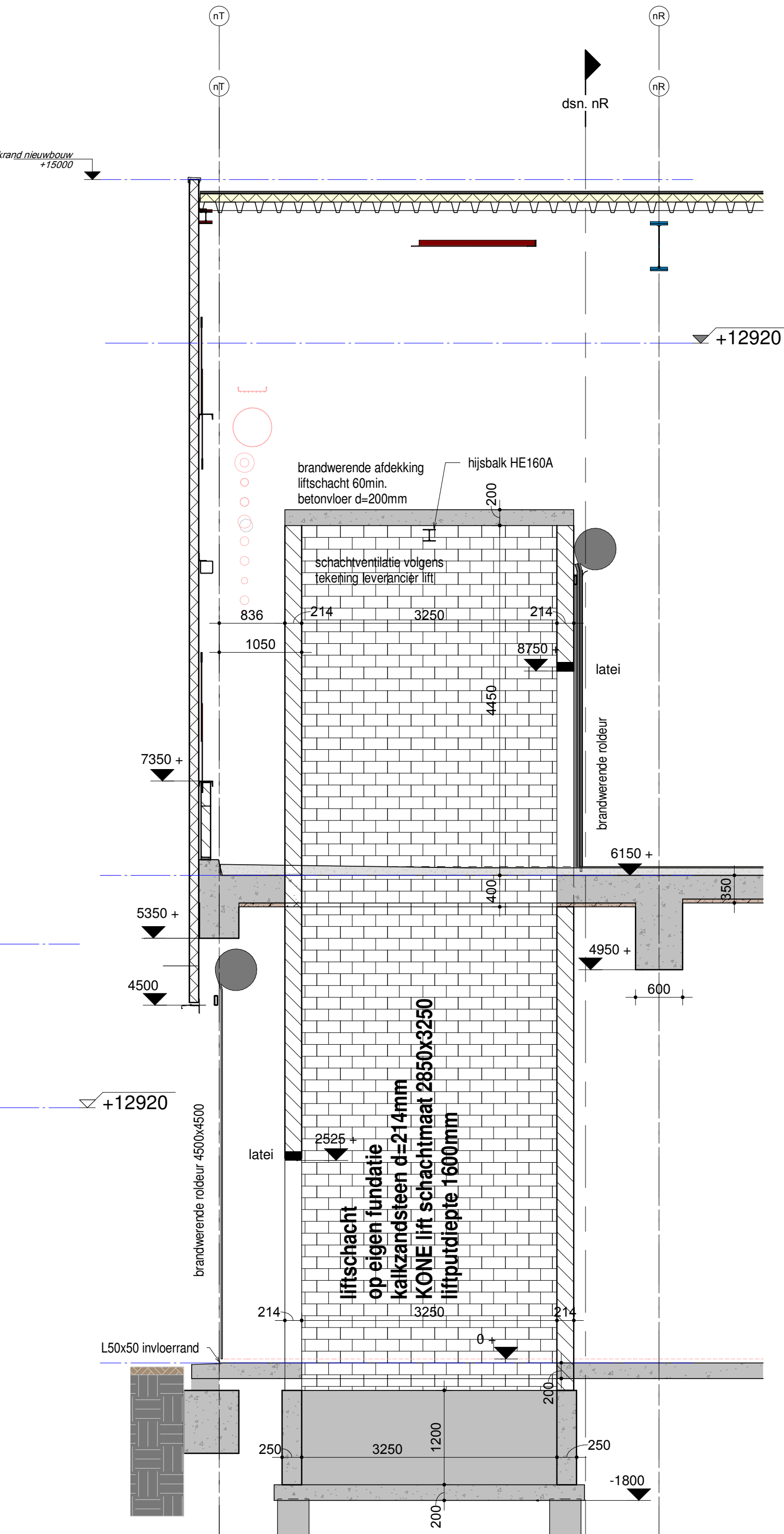
dsn. G12 (liftschacht) 1 : 50
