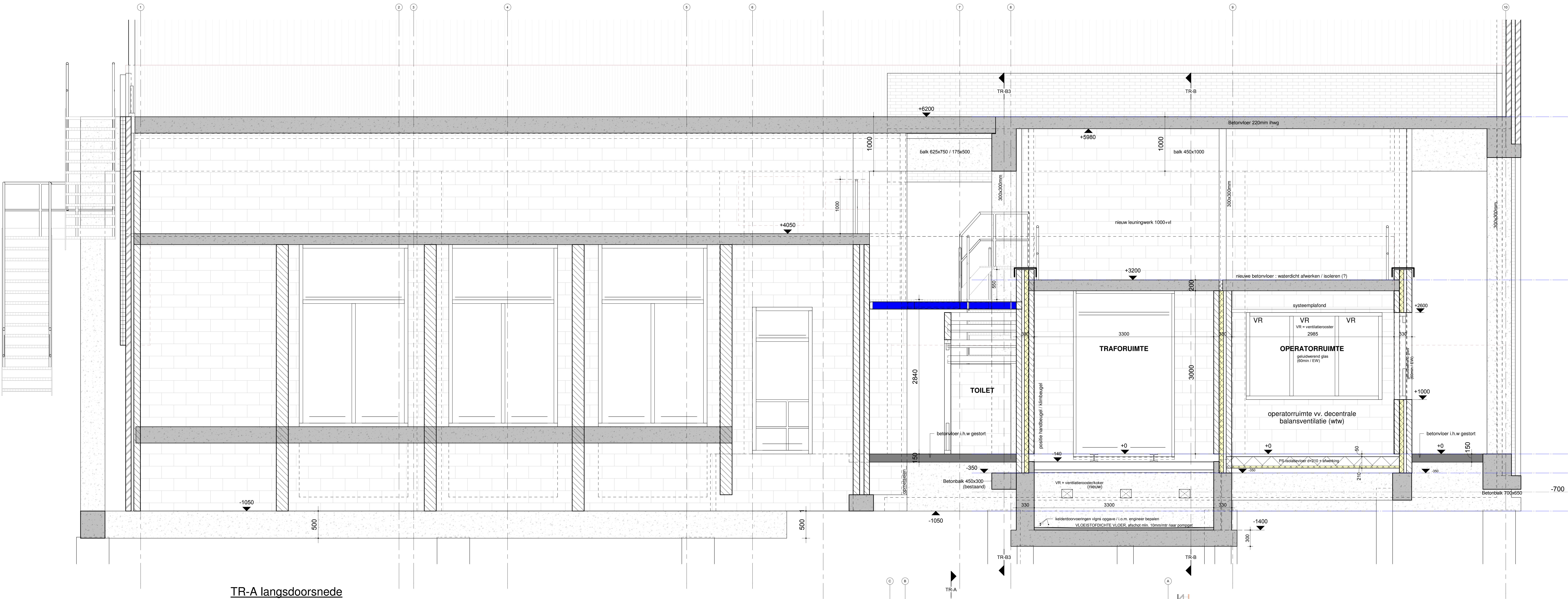
TR-A langsdoorsnede 1 : 25
