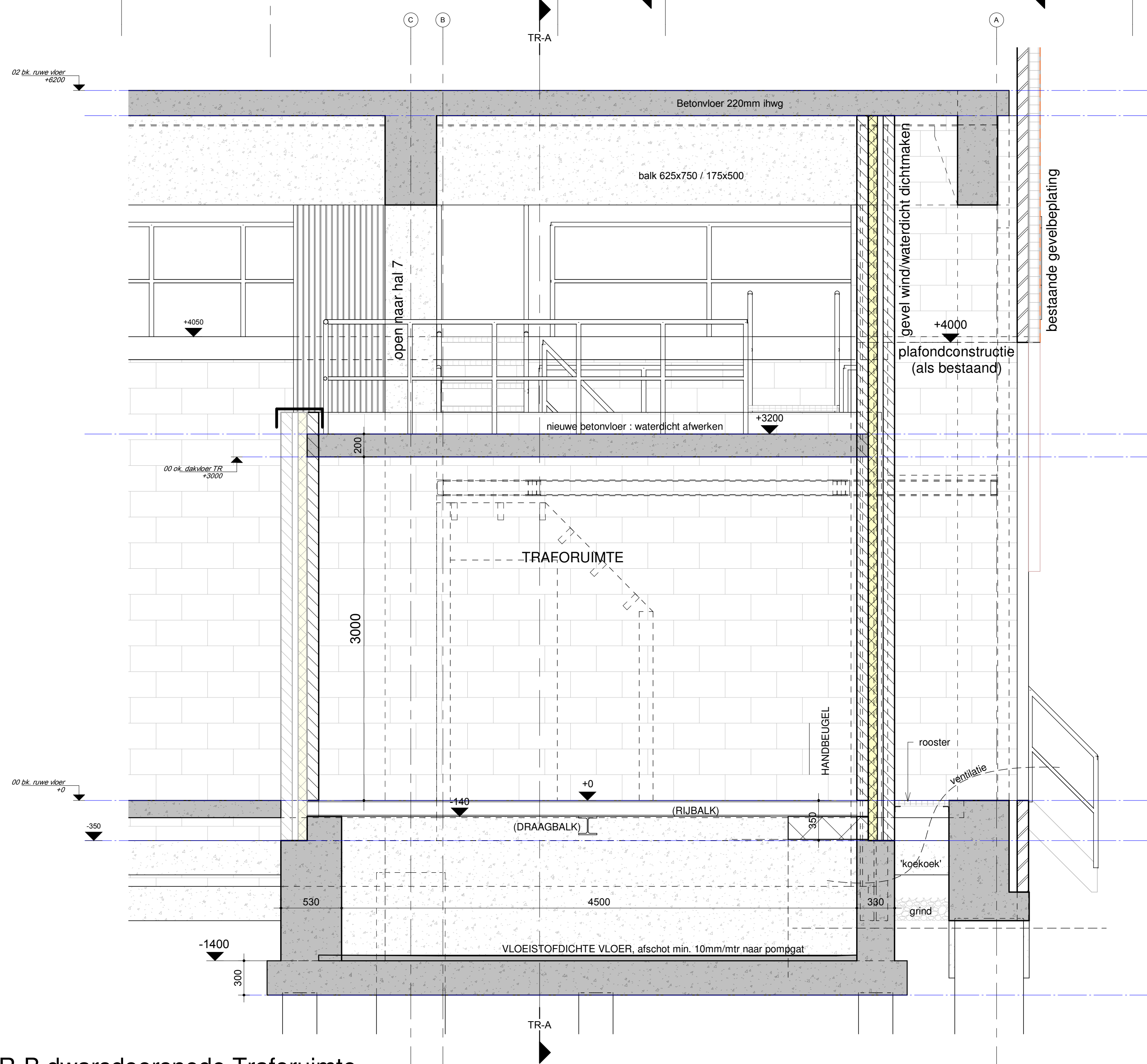
TR-B dwarsdoorsnede Traforuimte 1 : 25
