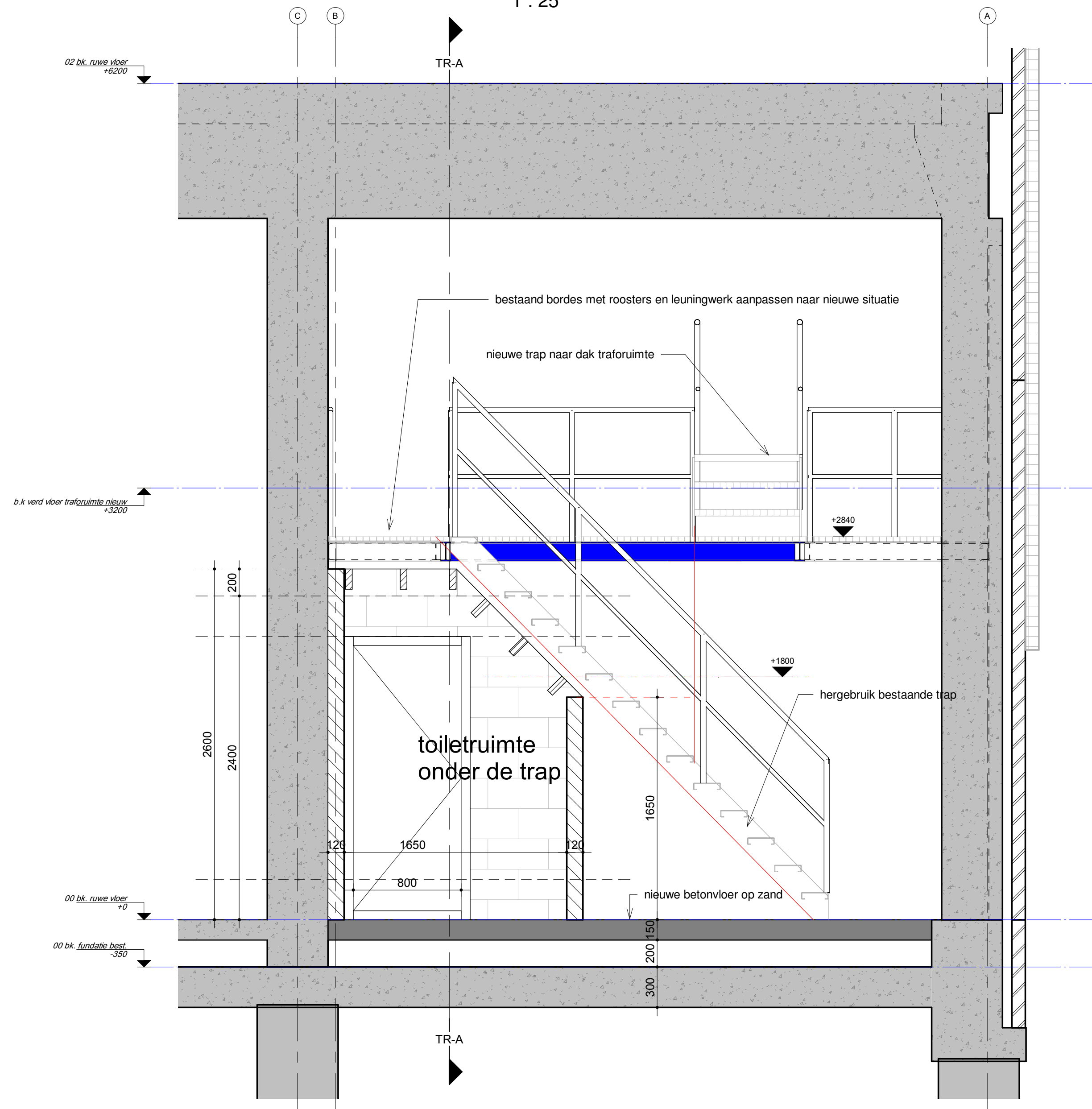
TR-B3 dwarsdoorsnede tpv toilettruimte en trap 1 : 25
