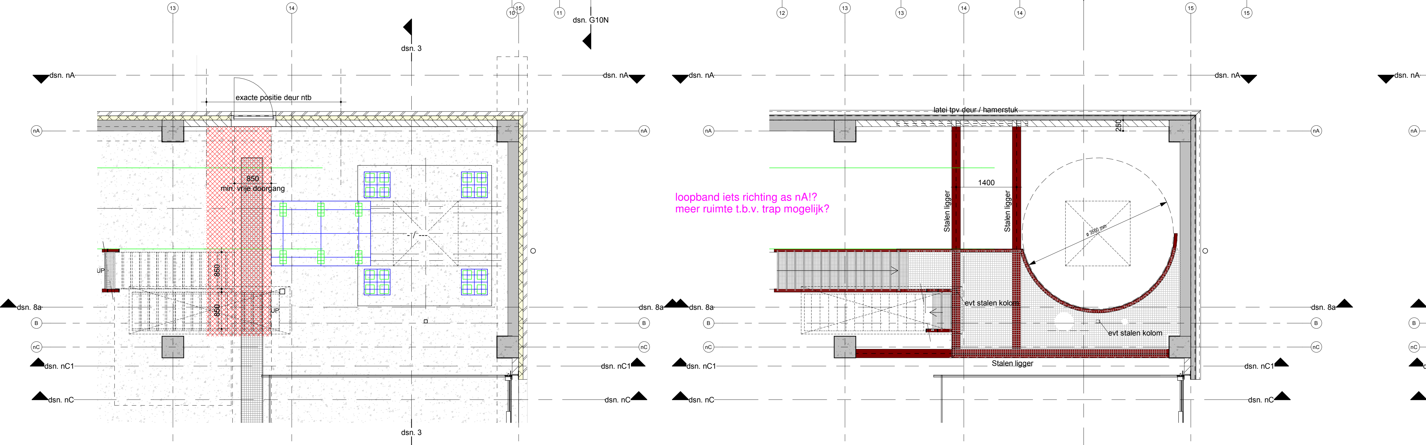
00 bk. ruwe vloer(3) pulper 1 : 50
