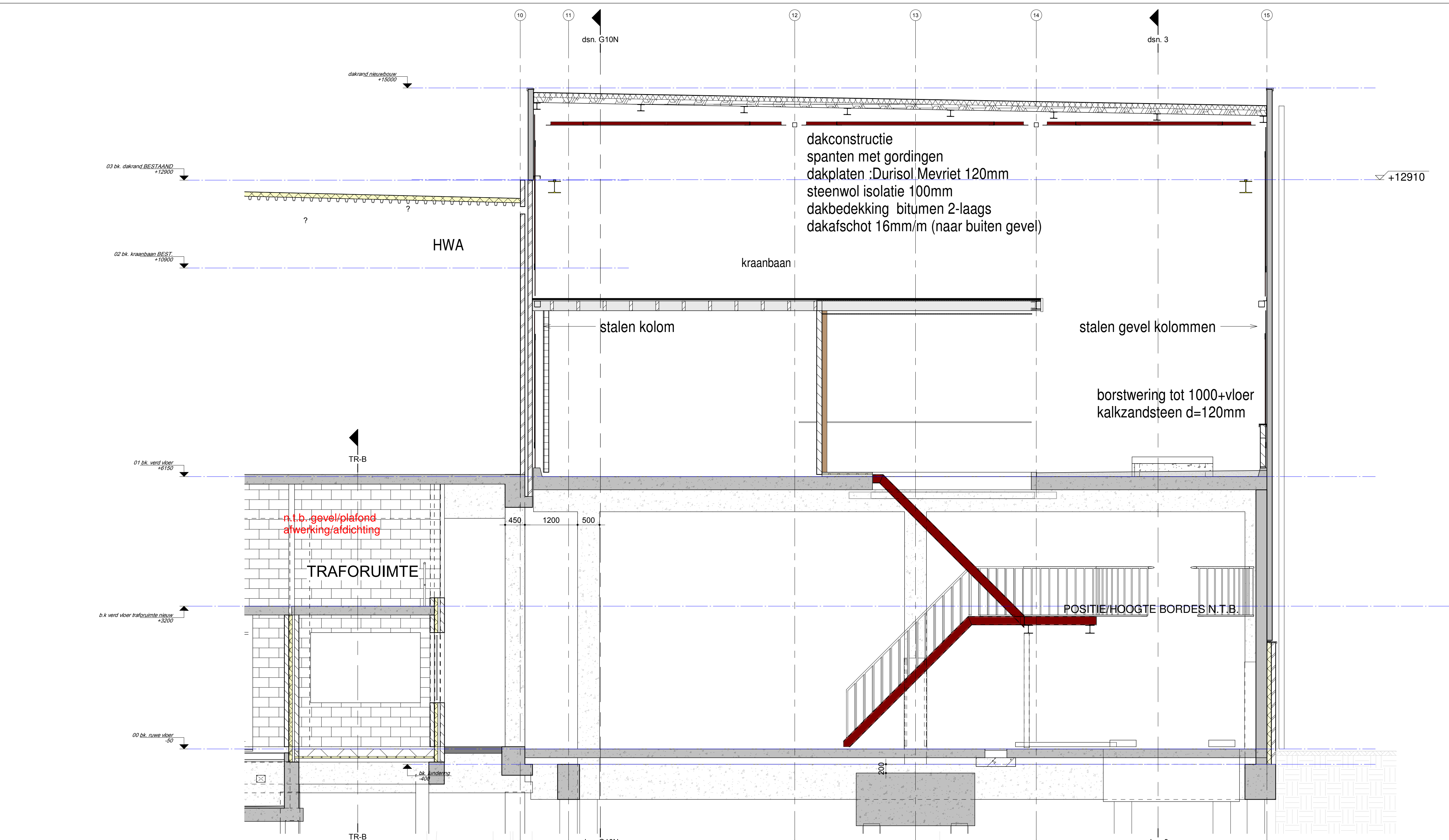
dwarsdoorsnede 8-8 1 : 50
