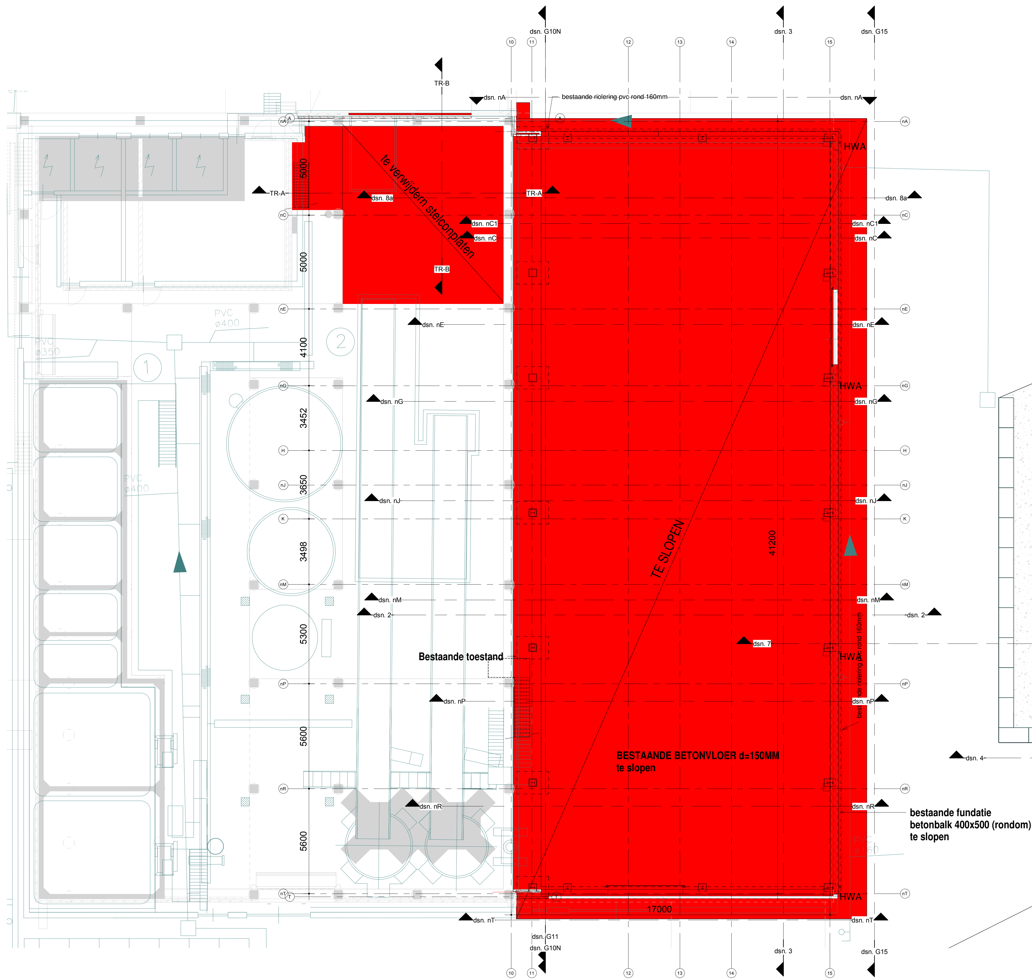
plattegrond bgg-vloer 1 : 100
