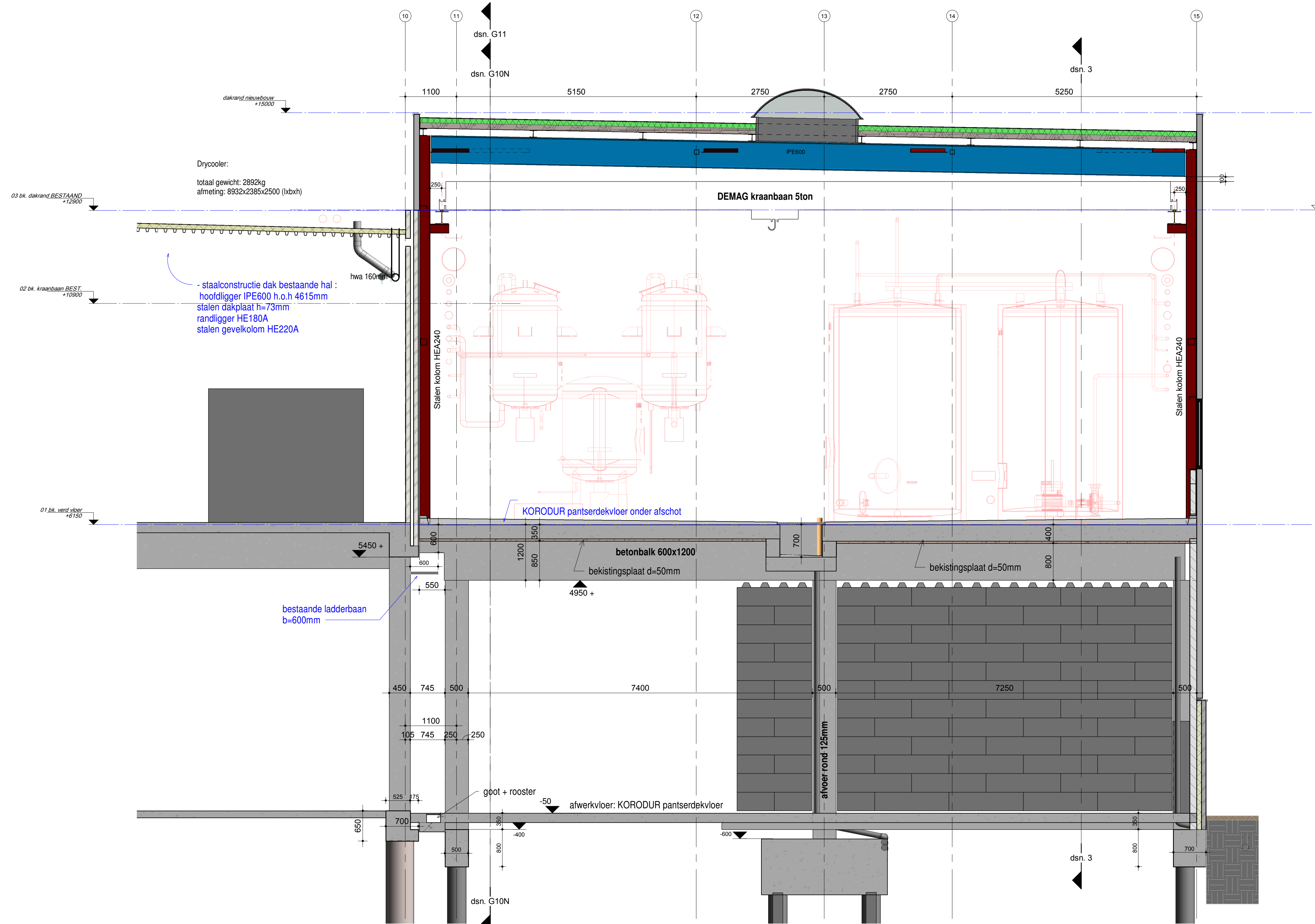
dsn. nG (stramien nG) 1 : 50
