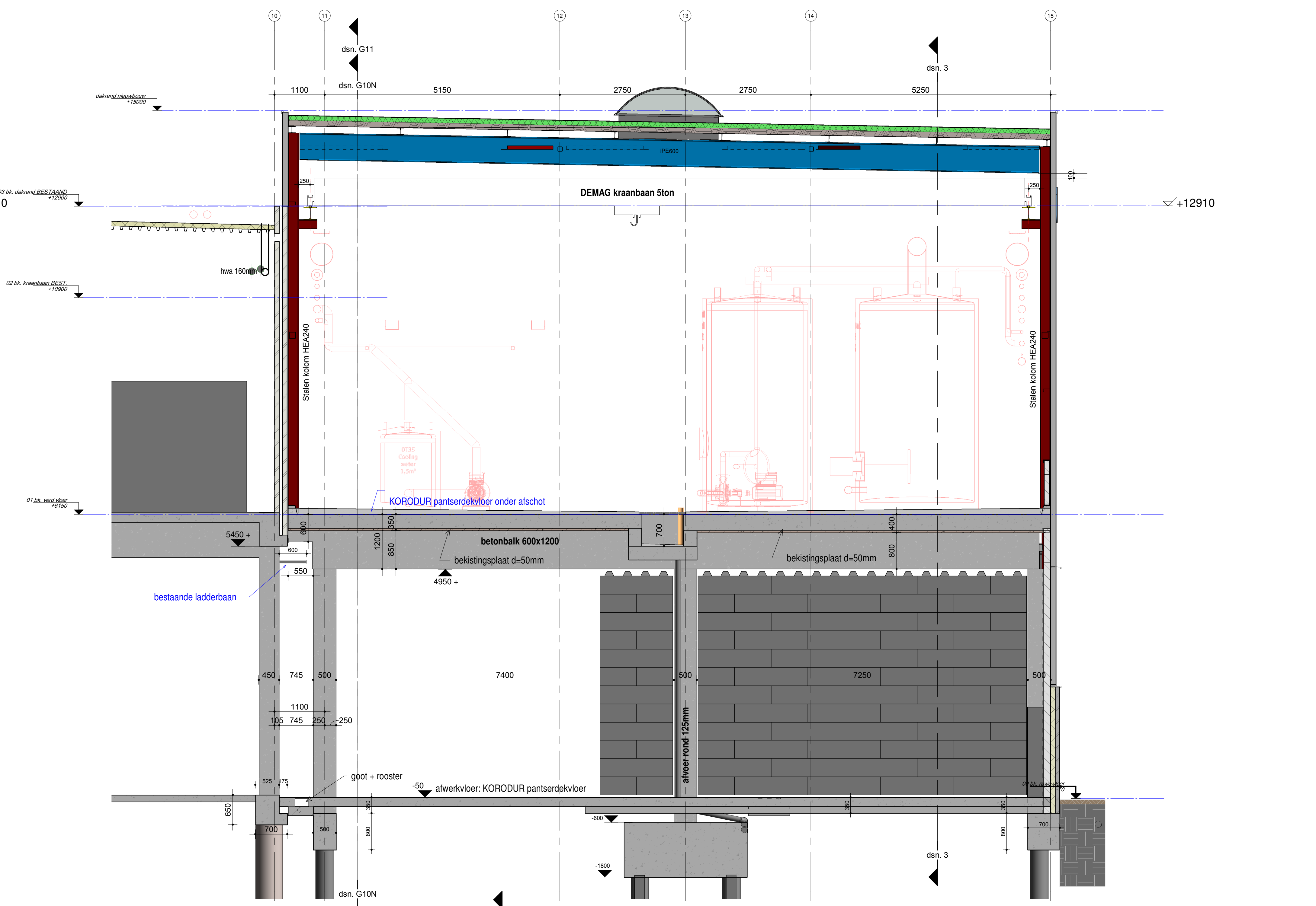
dsn. nE (stramien nE) 1 : 50
