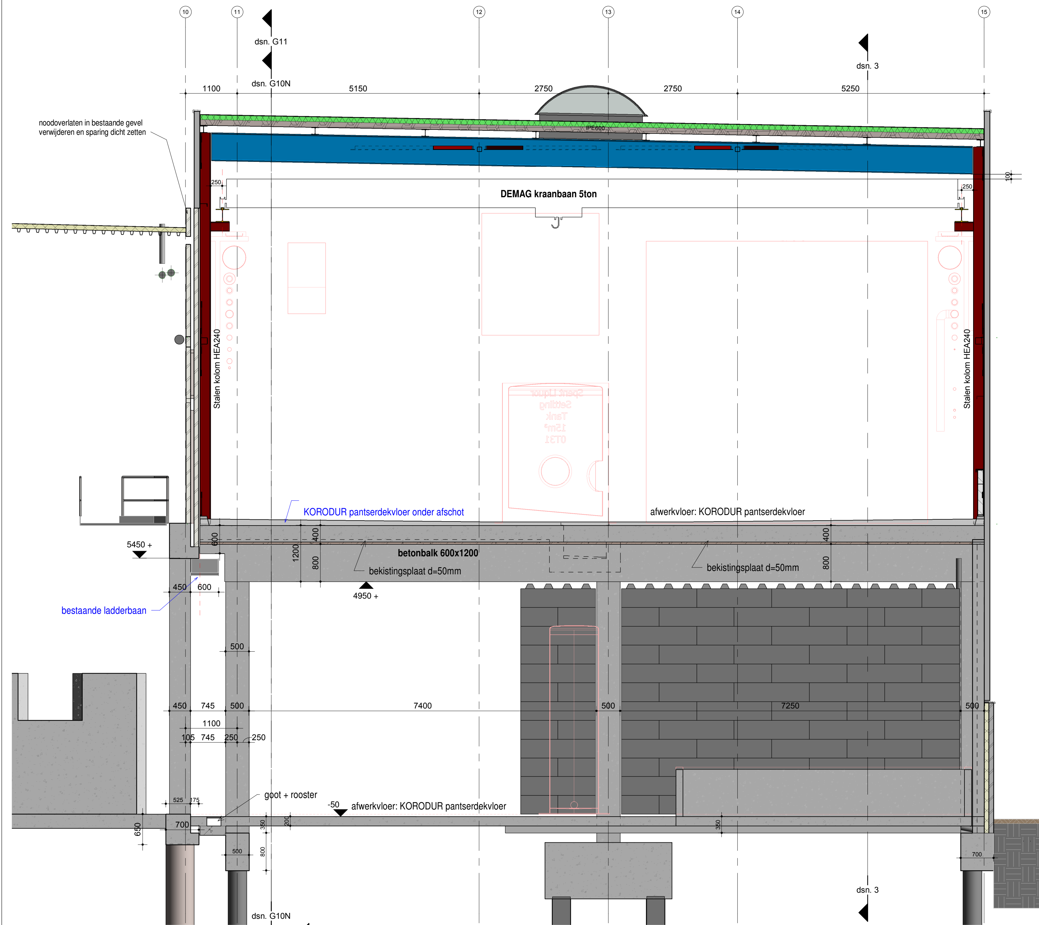
dsn. nR (stramien nR) 1 : 50
