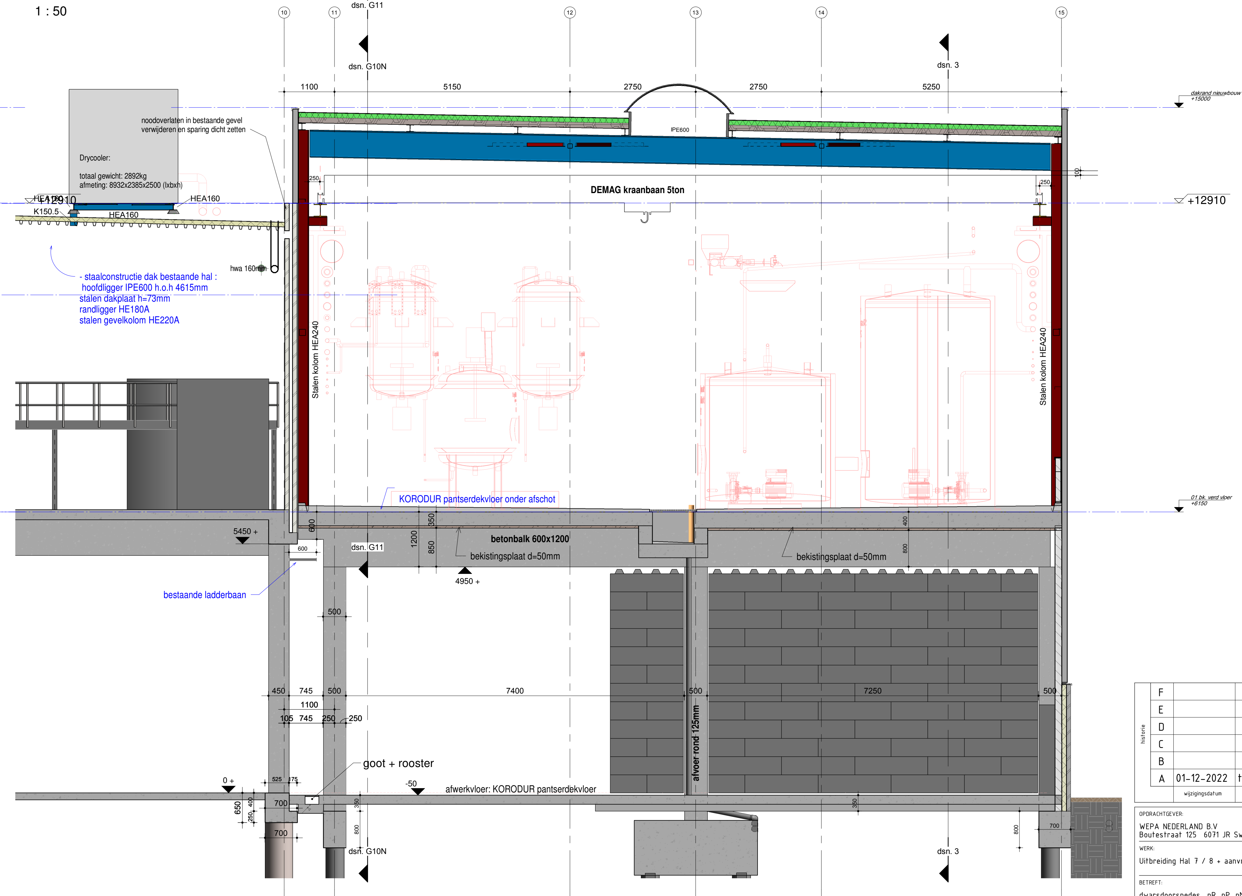
dsn. nJ (stramien nJ) 1 : 50
