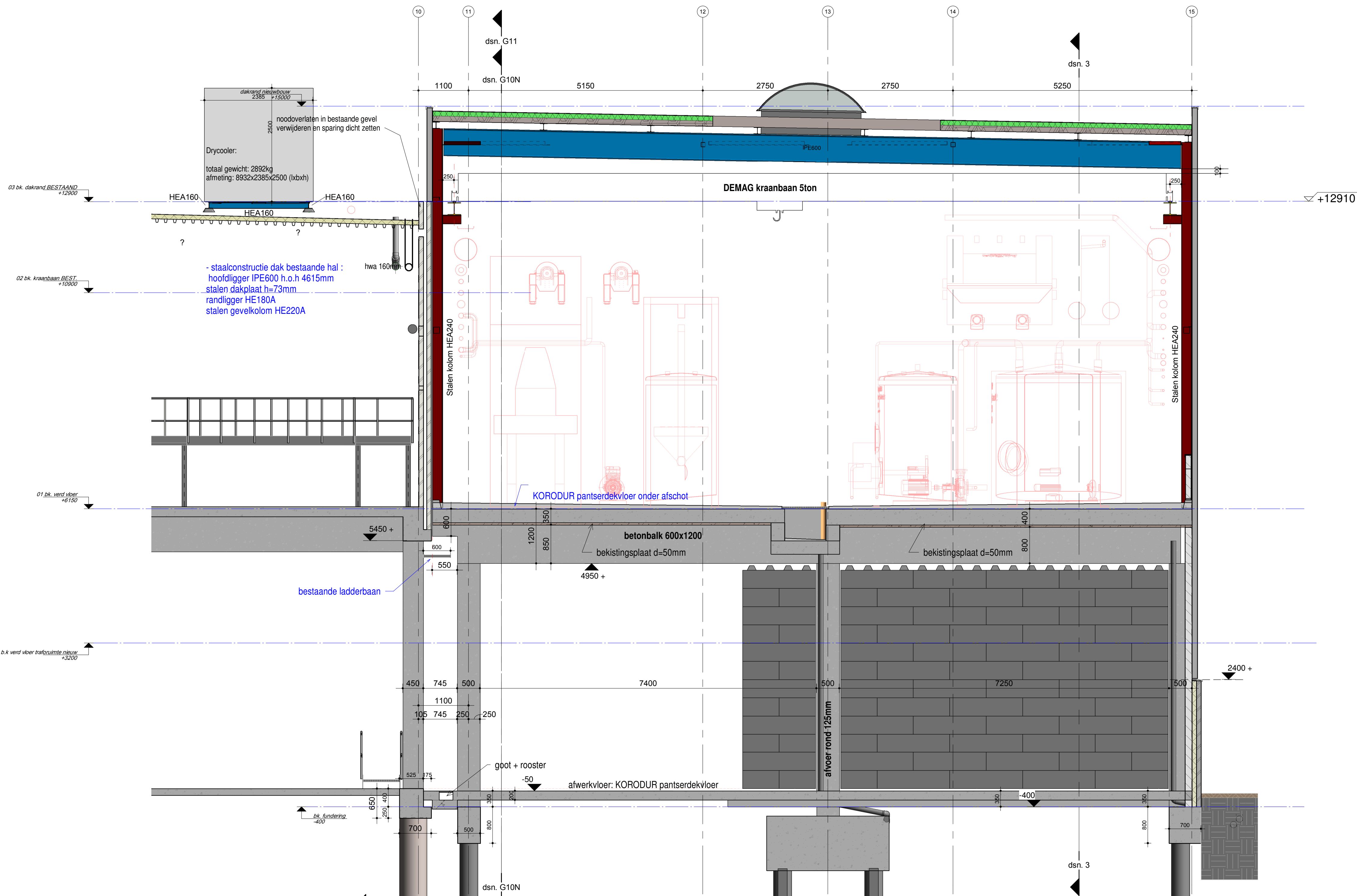
dsn. nM (stramien nM) 1 : 50
