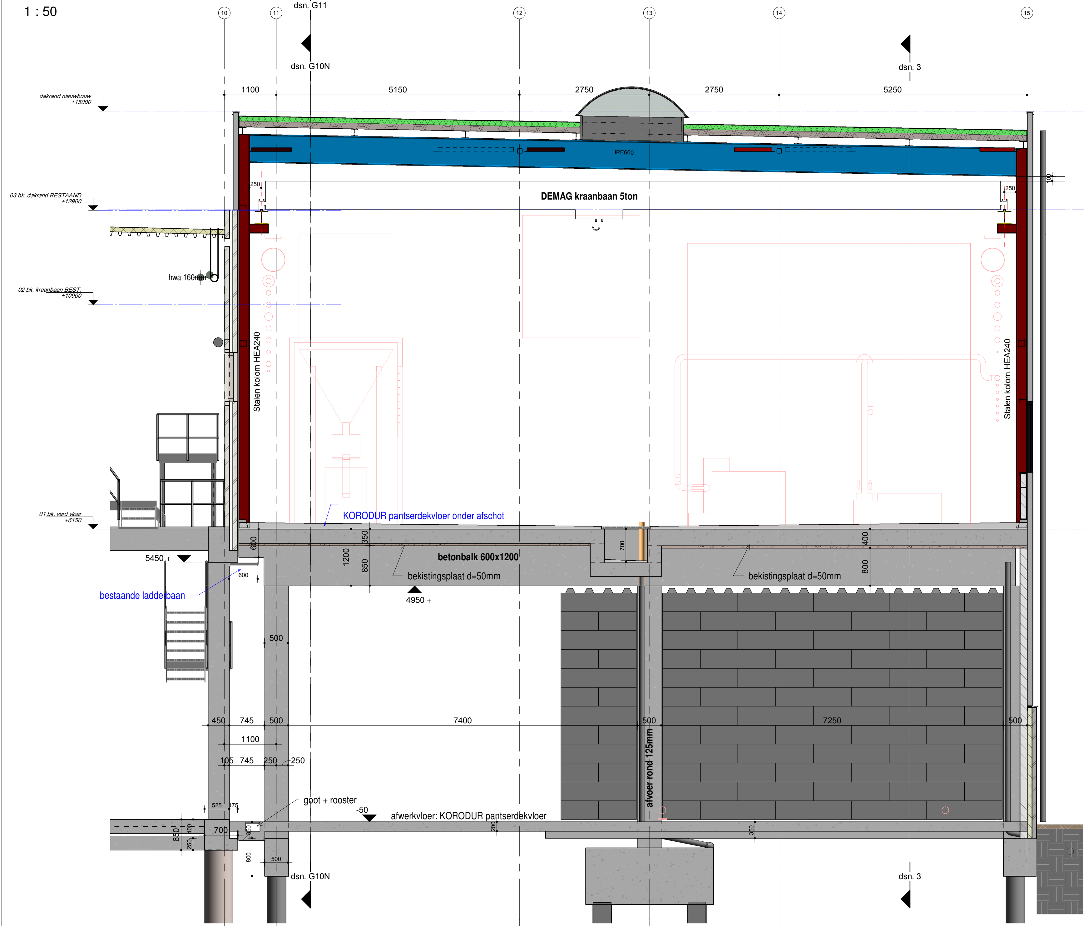
dsn. nP (stramien nP) 1 : 50
