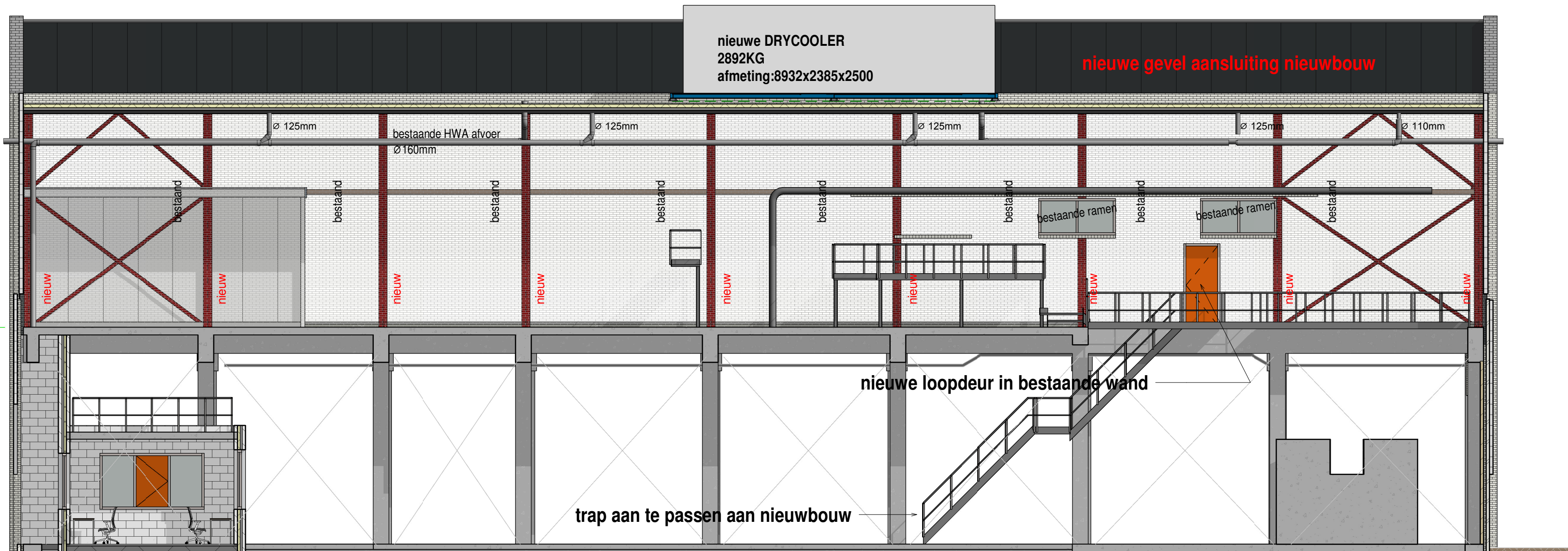
linkergevel (stramien 10 / 11 binnengevel)
