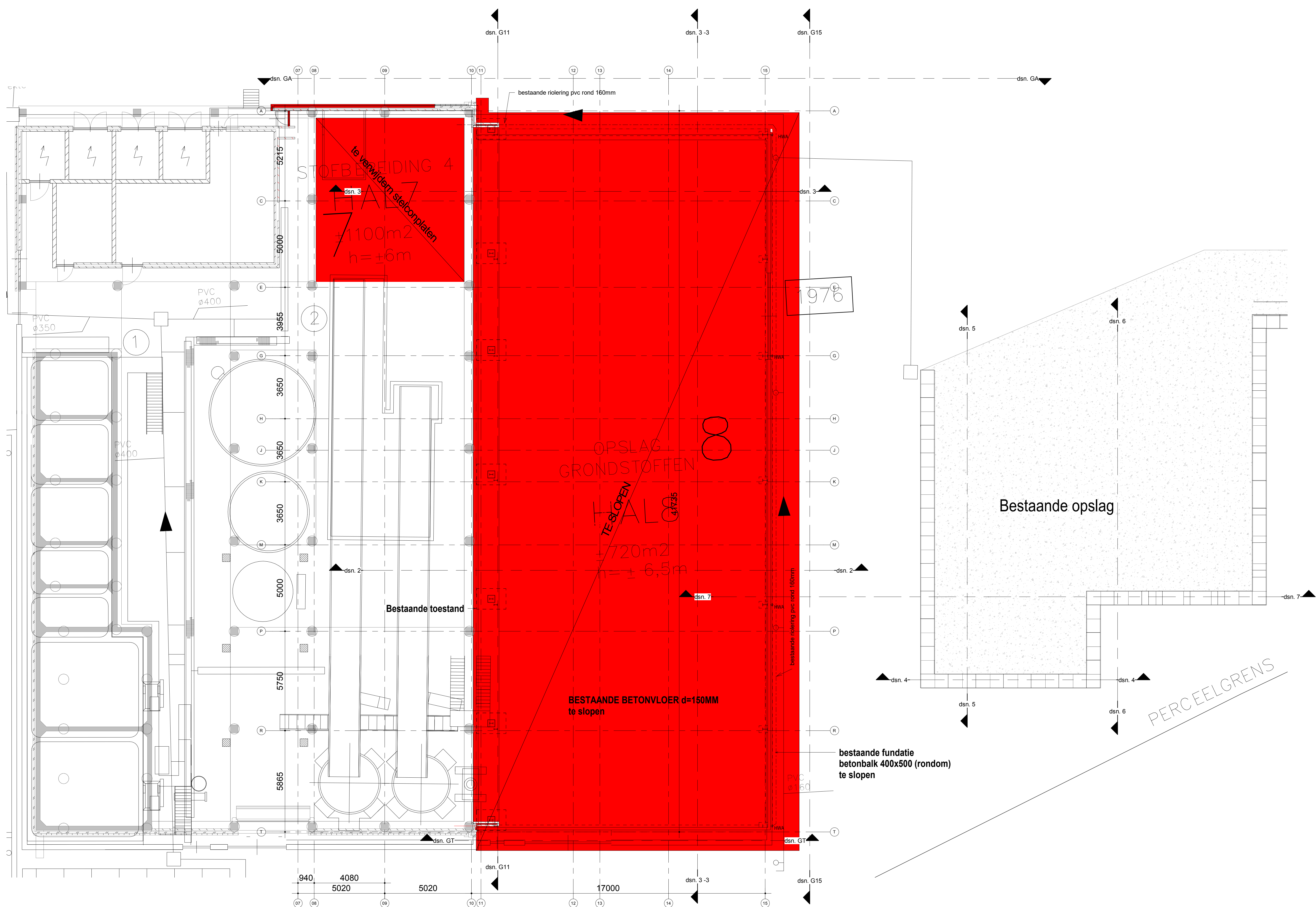
plattegrond bgg-vloer 1 : 100
