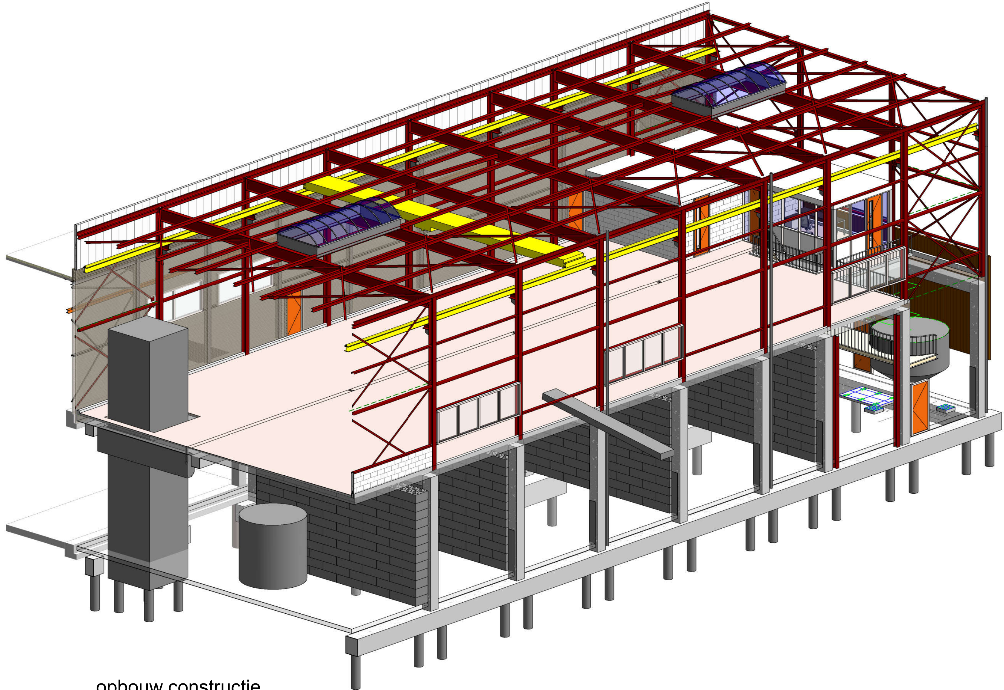
opbouw constructie
