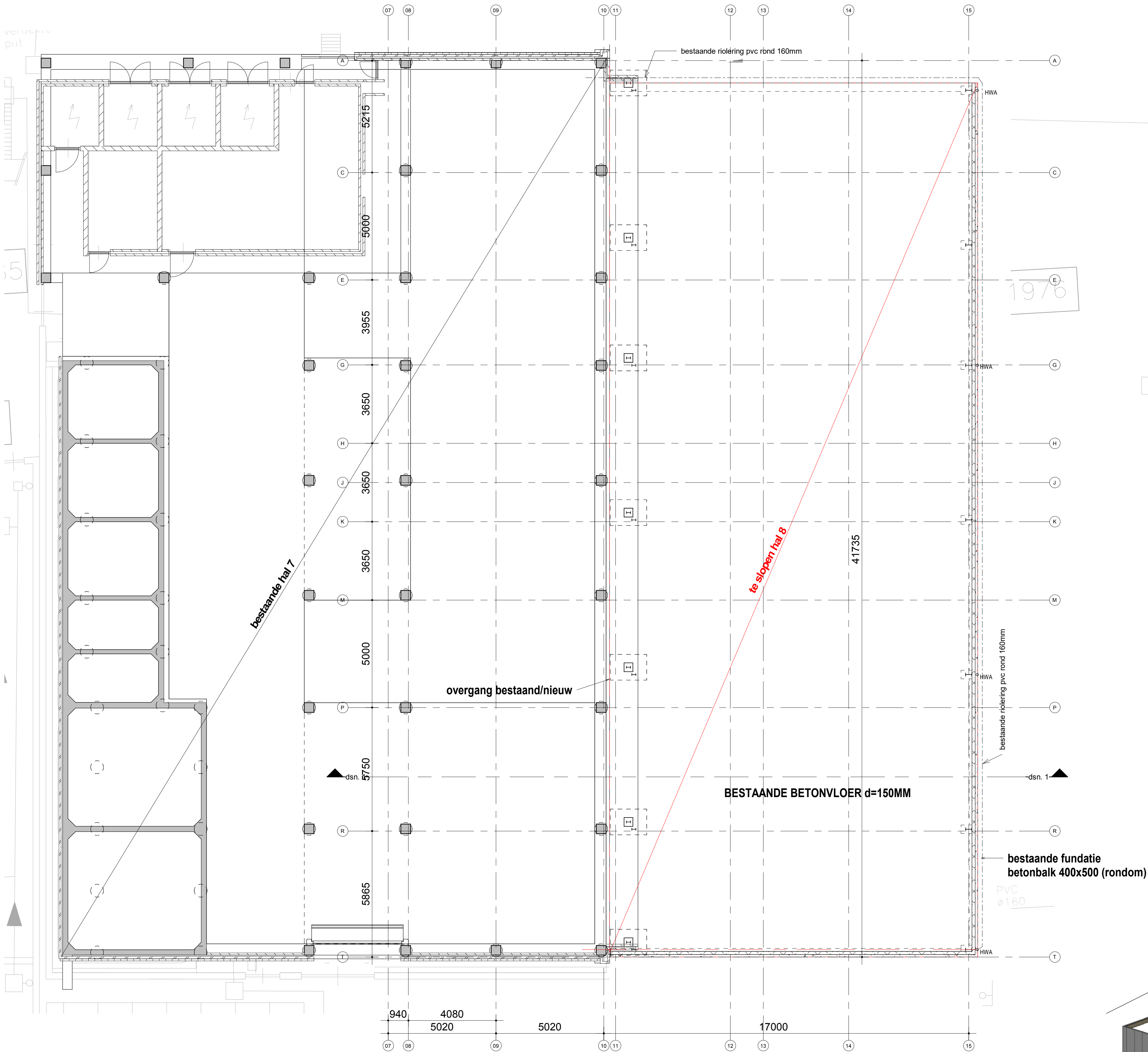
plattegrond bgg-vloer 1 : 100
