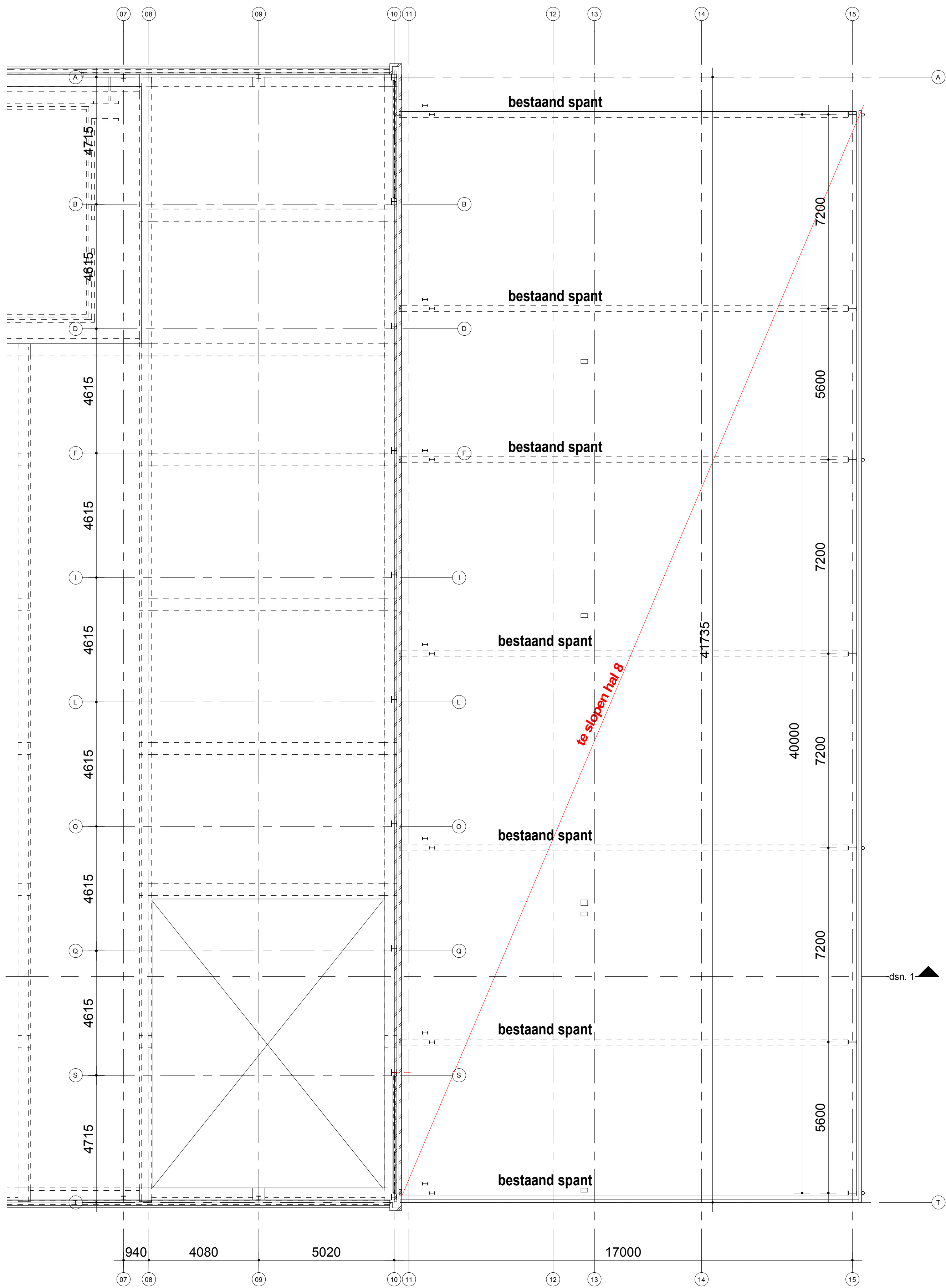
plattegrond op 6150+ 1 : 100
