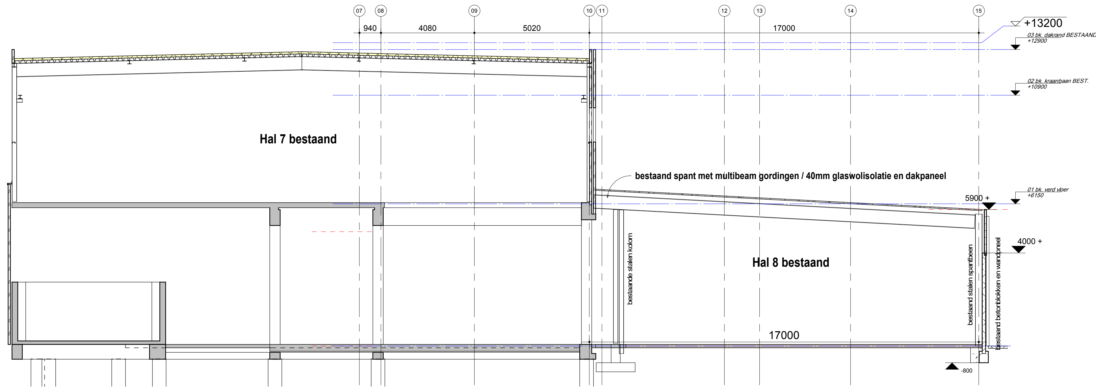
dsn. 1 - 1 (bestaande toestand) 1 : 100
