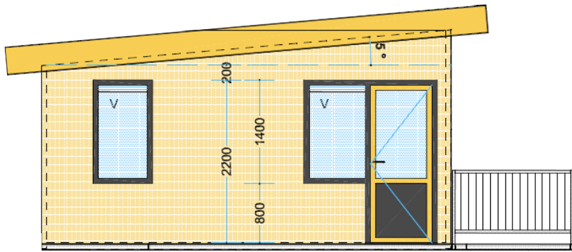
Zijaanzicht
