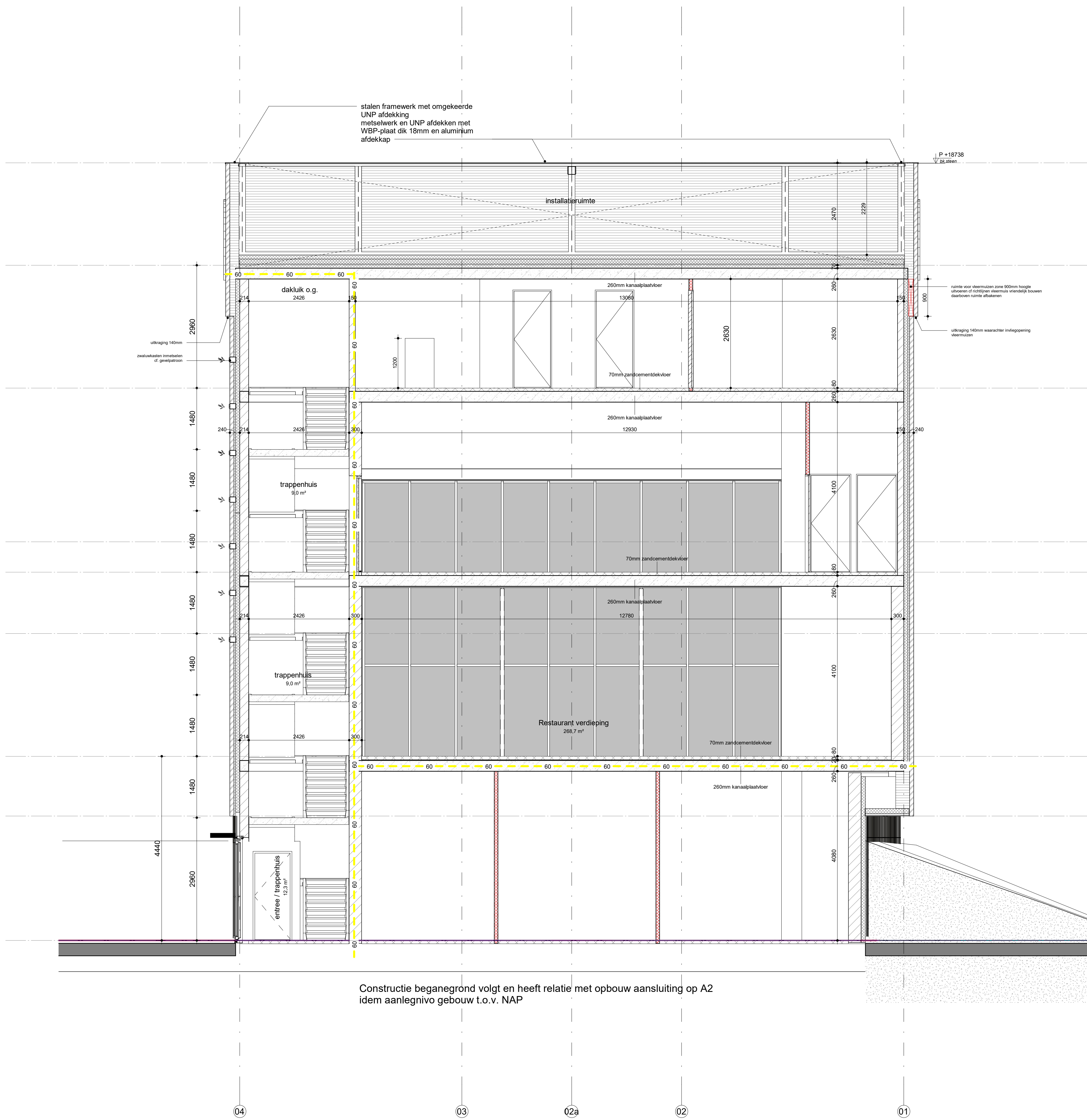
Doorsnede 1-1
