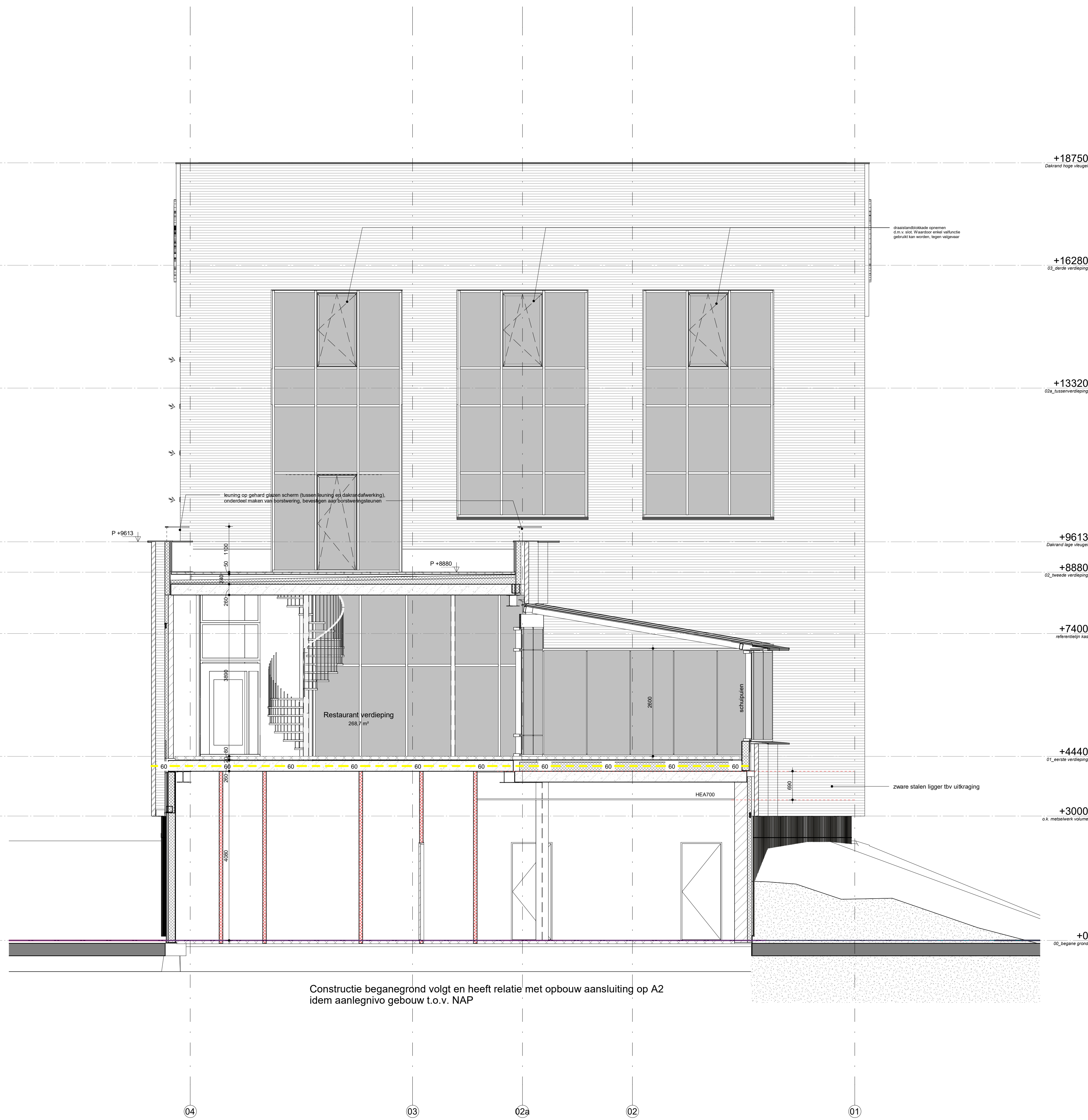
Doorsnede 2-2
