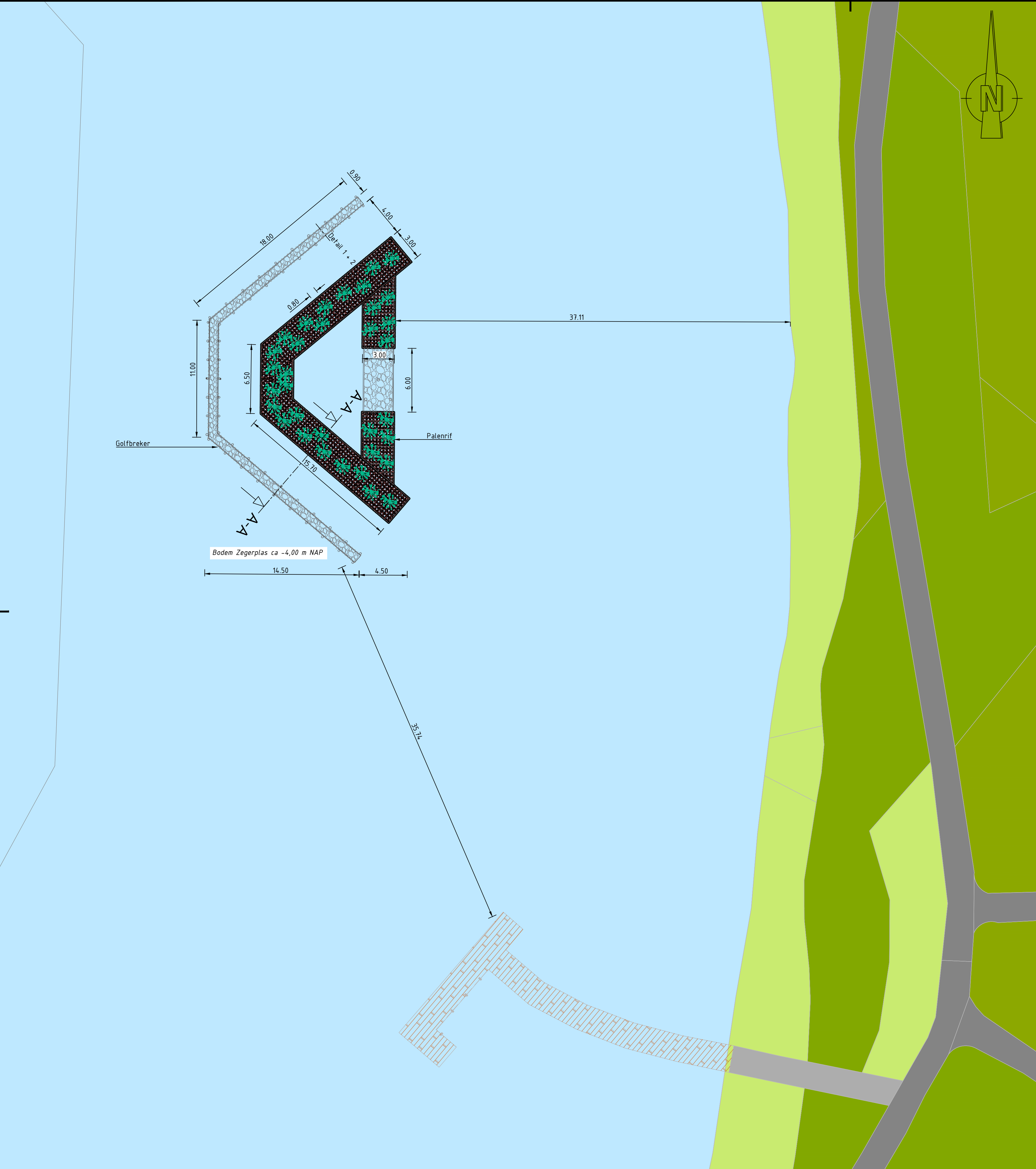
BOVENAANZICHT Schaal 1:200
