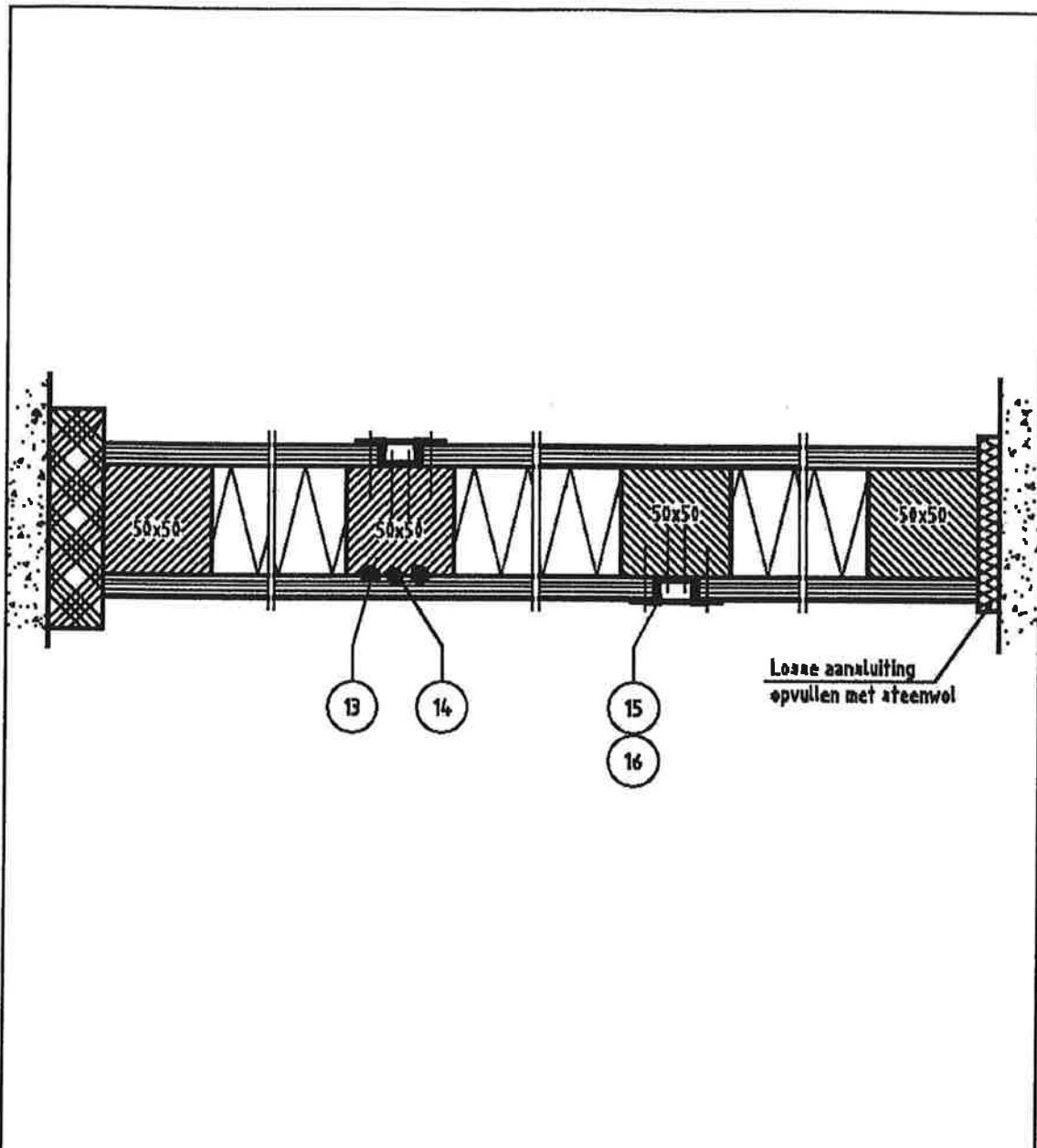
Figuur 1. Doorsnede wand, bovenaanzicht
