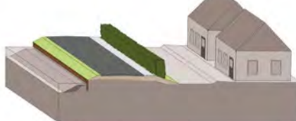
I 4b: Ophoging rijbaan
