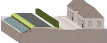
I 4a: Ophoging rijbaan i.c.m. bodemverzwaring
