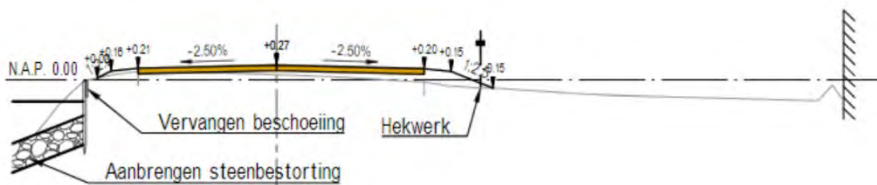
Figuur 17 Variant kruinophoging en bodemverzwarening
