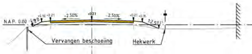
Figuur 27 Variant kruinophoging en bodemverzwaring
