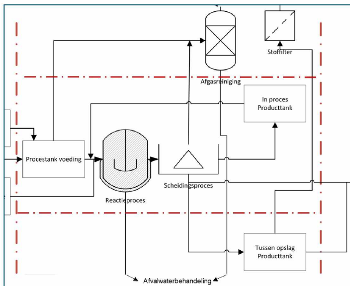
Figuur 5: schema productie organische vaste stoffen
