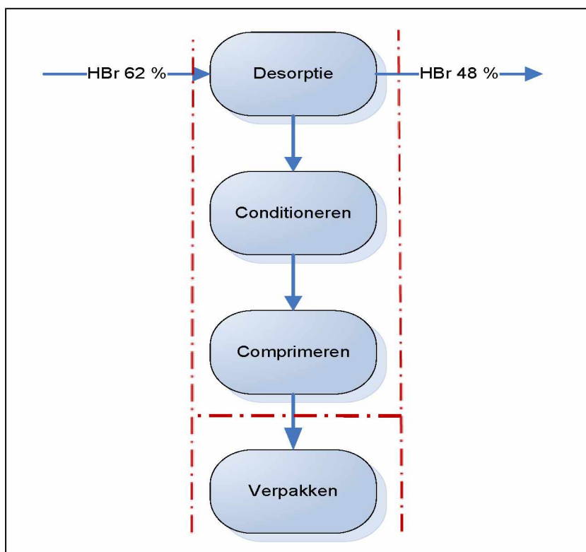
Figuur 3: schema productie anorganische gassen
