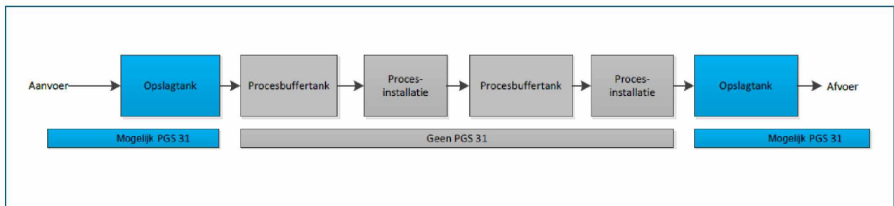
Figuur 1. Schematische weergave verschil opslagtank en proces tank
