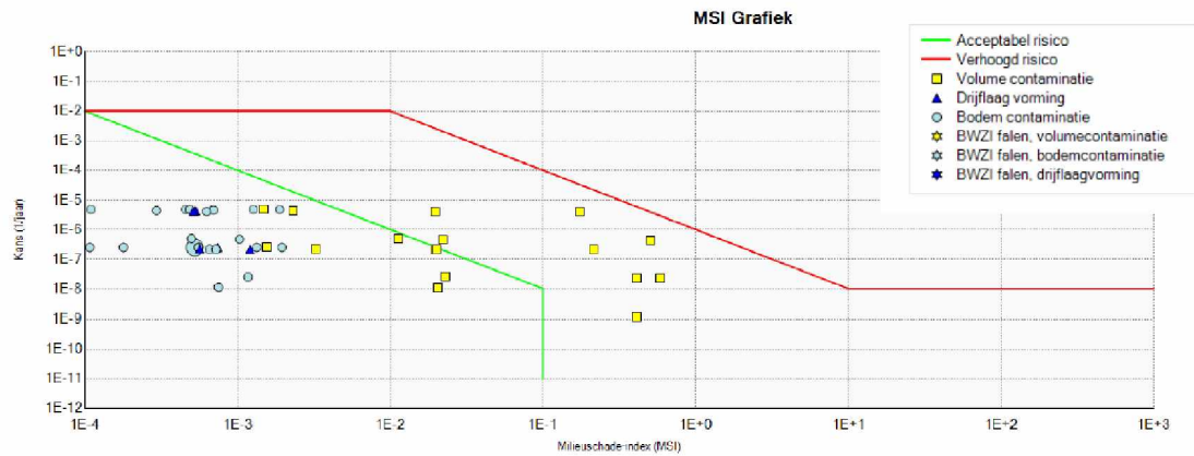
Figuur 0.4 – MSI grafiek Proteus File "GBC West" (Bijlage 7)
