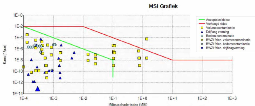
Figuur 0.3 – MSI grafiek Proteus File "Solids 5 West (inclusief Broomhandling en stukgoedopslag)" (Bijlage 7)
