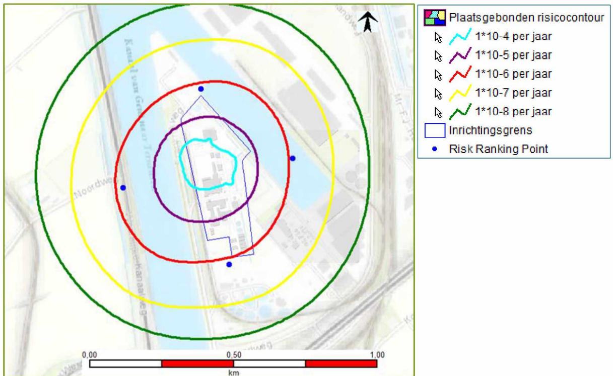
Figuur 0.1 – Berekende plaatsgebonden risicocontouren ICL-IP Terneuzen (bijlage 6)
