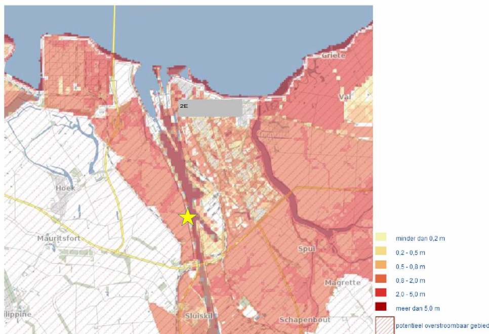
Figuur 1.13: Overstroombaar gebied en maximale waterdiepte bij kleine kans op overstromen, waarbij de gele ster de locatie van ICL-IP aangeeft (Bron: nederland.overstromingsrisicokaart.nl).
