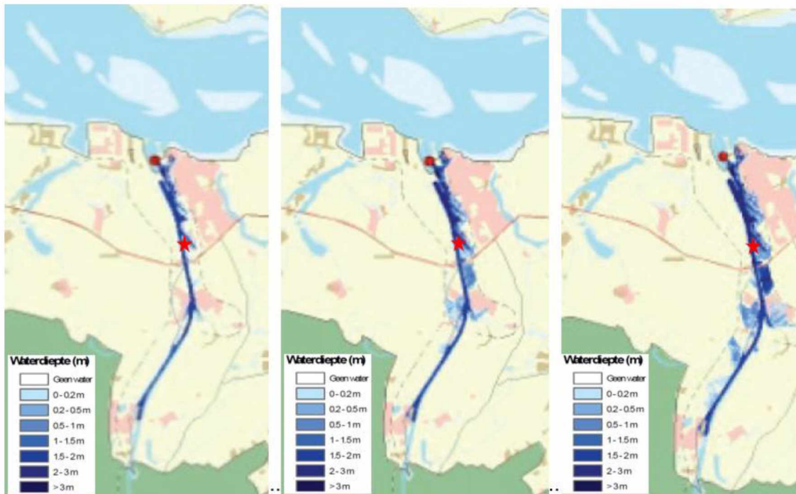
Figuur 1.14: Maximale waterdiepte bij dijkdoorbraak ringdeel 20. Rode ster geeft locatie ICL-IP weer (Bron: VNK2). Links: overstroming met buitenwaterstand die met een kans van 1/40.000 per jaar voorkomt. Midden: overstroming met buitenwaterstand die met een kans van 1/40.000 per jaar voorkomt waarbij alle sluisdeuren falen. Rechts: overstroming met buitenwaterstand die met een kans van 1/400.000 per jaar voorkomt.
