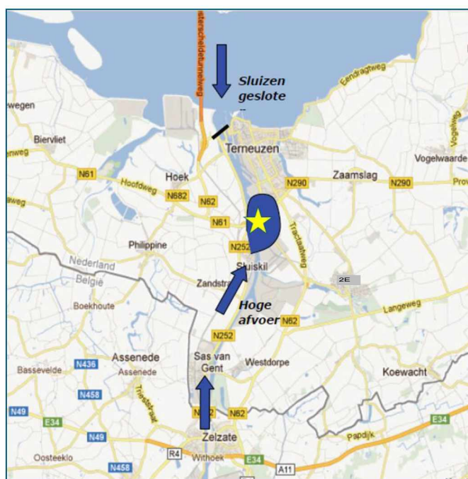
Figuur 1.12: Schematisch beeld van mogelijk overstrooming bij gesloten sluisen bij Terneuzen en een hoge afvoer vanuit België. Gearceerd deel scenario betreft een illustratie van een mogelijk overstroomingsscenario op een willekeurige locatie. De gele ster geeft de locatie van ICL-IP weer. (Bron: VNK, dijkkringgebied 32).
