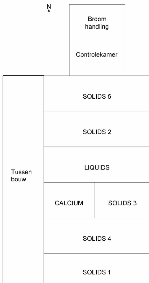
Figuur 2.1 Bovenaanzicht GBC-gebouw
