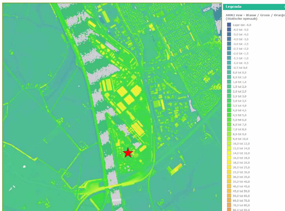
Figuur 1.11: Maaiveldhoogtes in de omgeving van ICL-IP Terneuzen. Locatie is aangeduid met rode ster (bron: AHN2).
