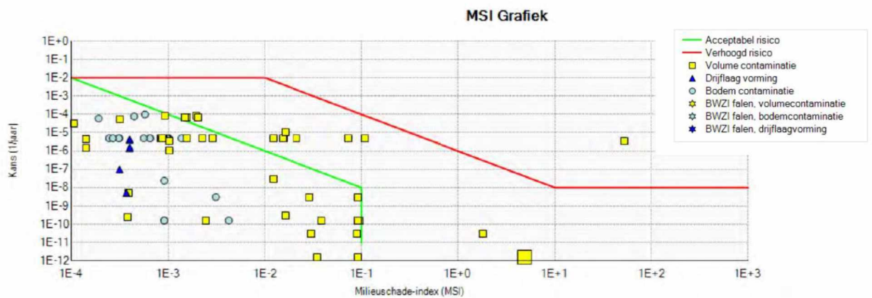
Figuur 0.5 – MSI grafiek Proteus File "GBC-Oost HBr BRU 4in1 Leidingwerk" (Bijlage 7)
