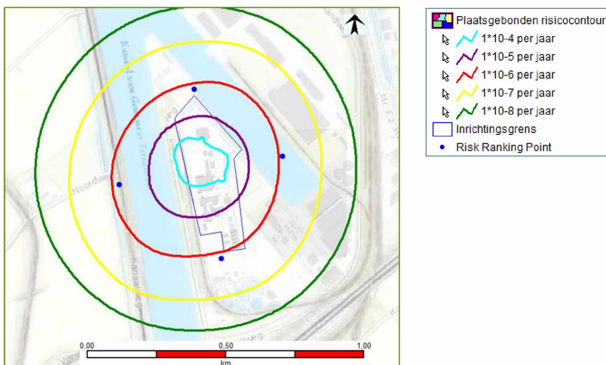
Figuur 4.4. Plaatsgebonden risicocontouren Safeti-NL versie 8.21 [5]
